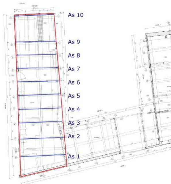
Afb. 76: Assensysteem schuur.
