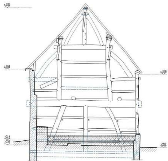
Afb. 74: Origineel eindspant op as 6.
