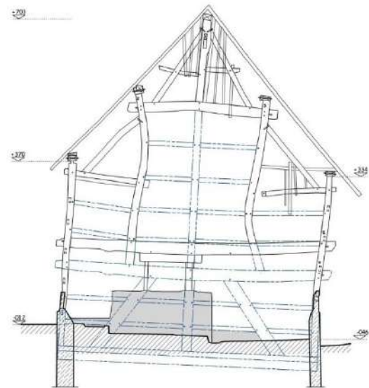
Afb. 86: Oorspronkelijk eindspant op as 3.
