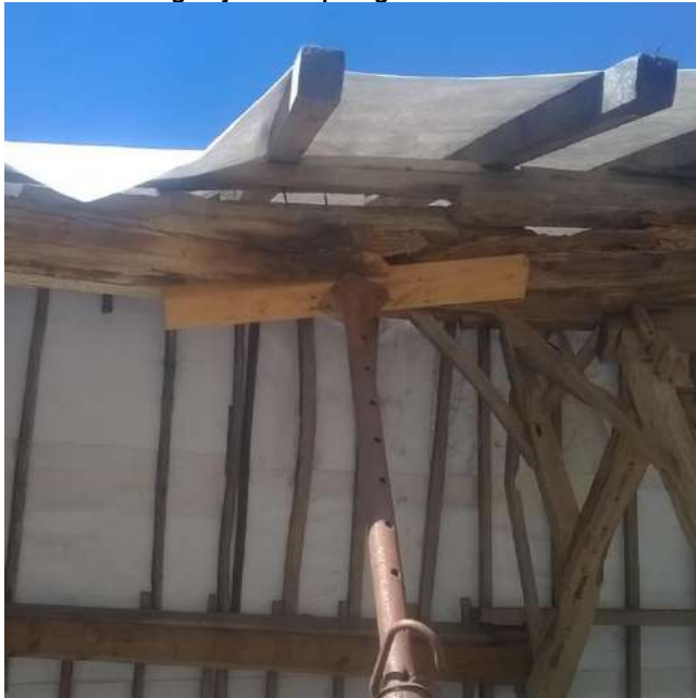
Afb. 77: Gestut vakwerk schuur.
