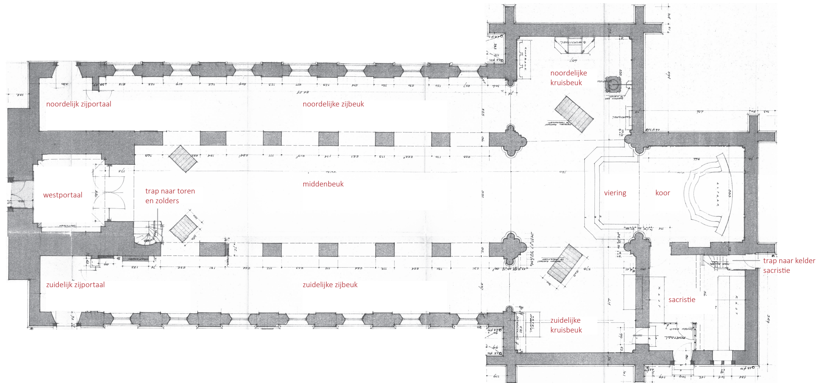
Afb. 106. Grondplan van de Sint-Pieterskerk met nomenclatuur van de bouwdeelen.
