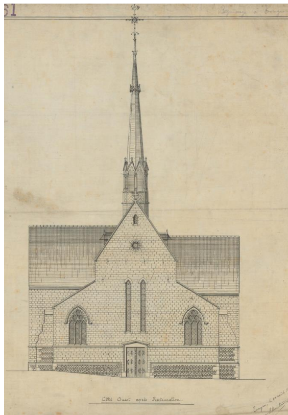
Plan restauratie begijnhofkerk Christiaens – westgevel (1894) en plan restauratie begijnhofkerk Christiaens – noordgevel (1894)
