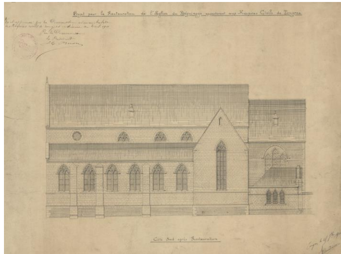
Plan restauratie begijnhofkerk Christiaens – zuidgevel na restauratie (1901) en plan restauratie begijnhofkerk Christiaens – westgevel en oostgevel na restauratie (1901).
