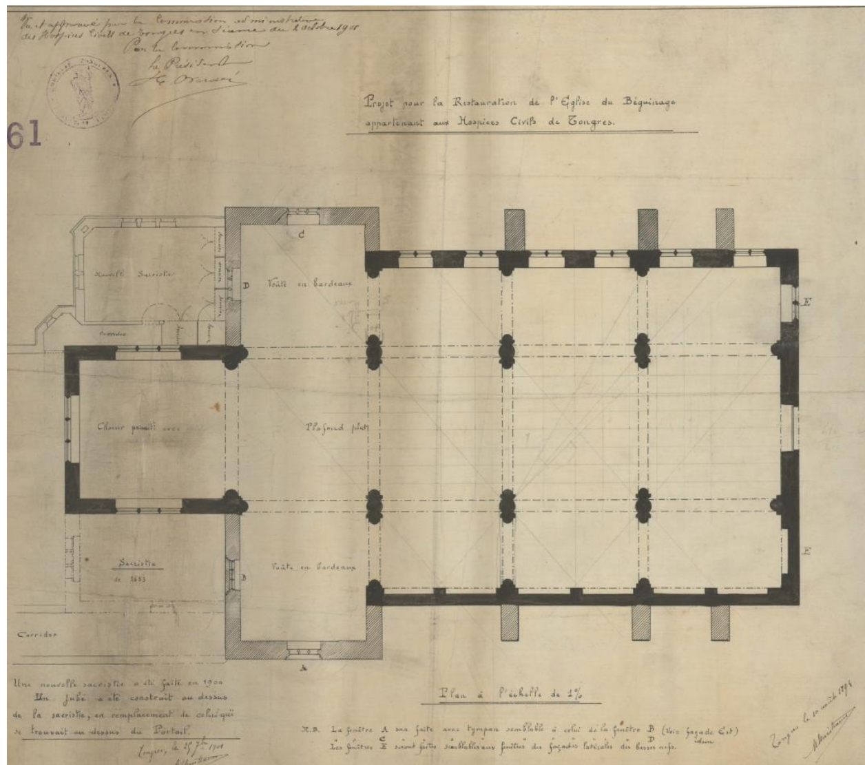
Plan restauratie begijnhofkerk Christiaens – grondplan (1894)
