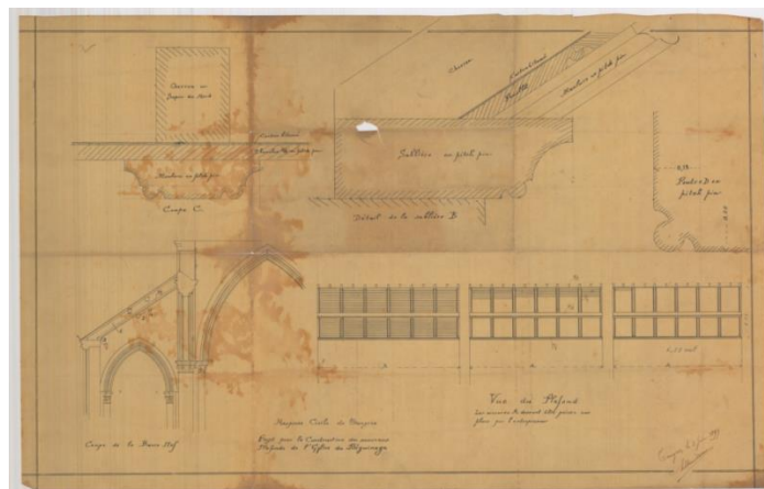
Plan restauratie plafond, 1899 (architect Mathieu Christiaens) (SAT, kaarten en plannen, 126)
