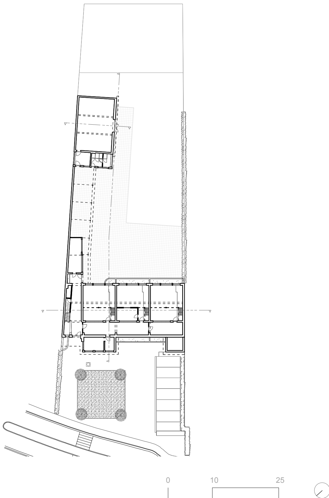
Bestaande plannen - inplantingsplan
