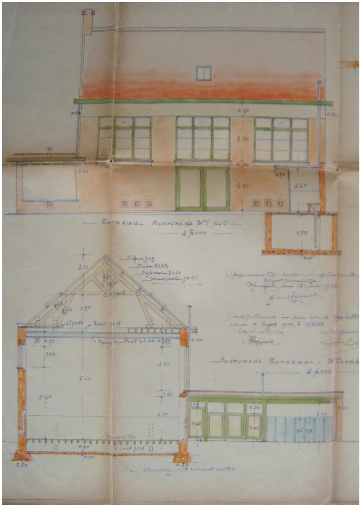
Originele tekening - turnzaal
