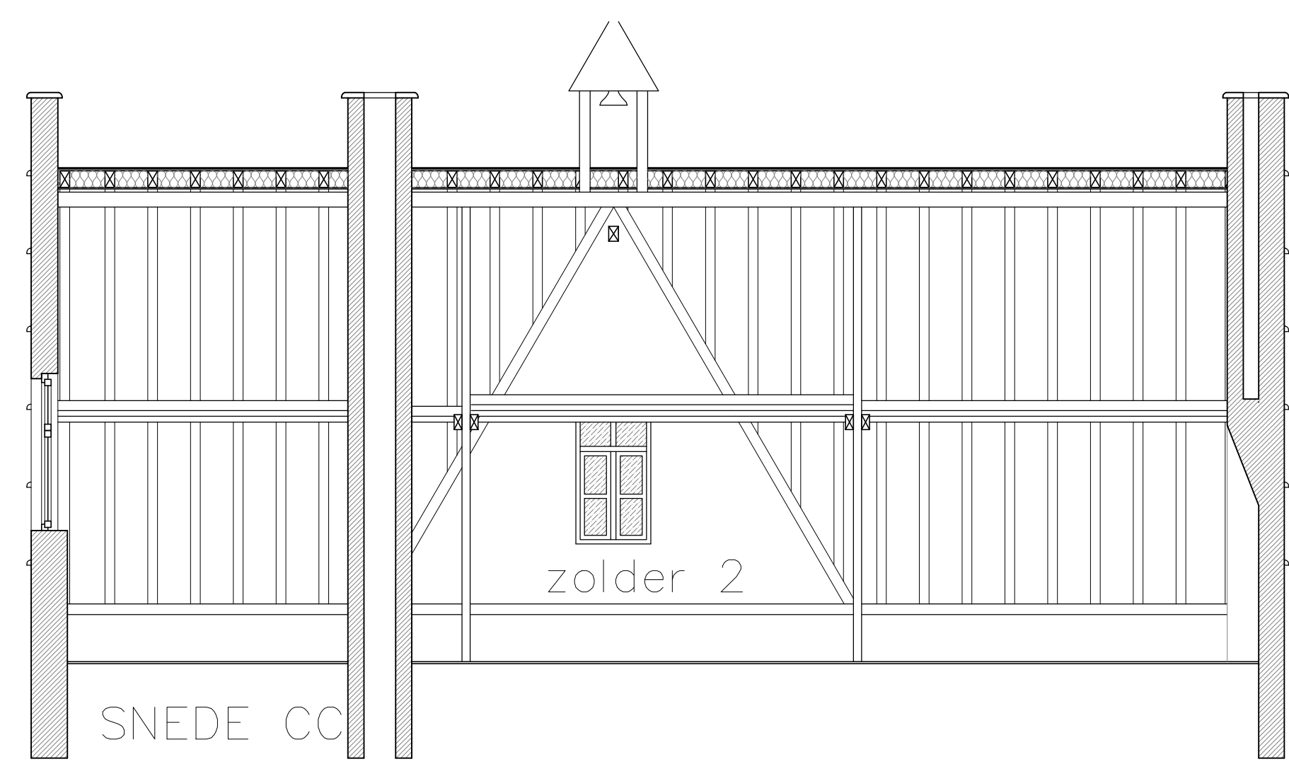
SNEDE CC
