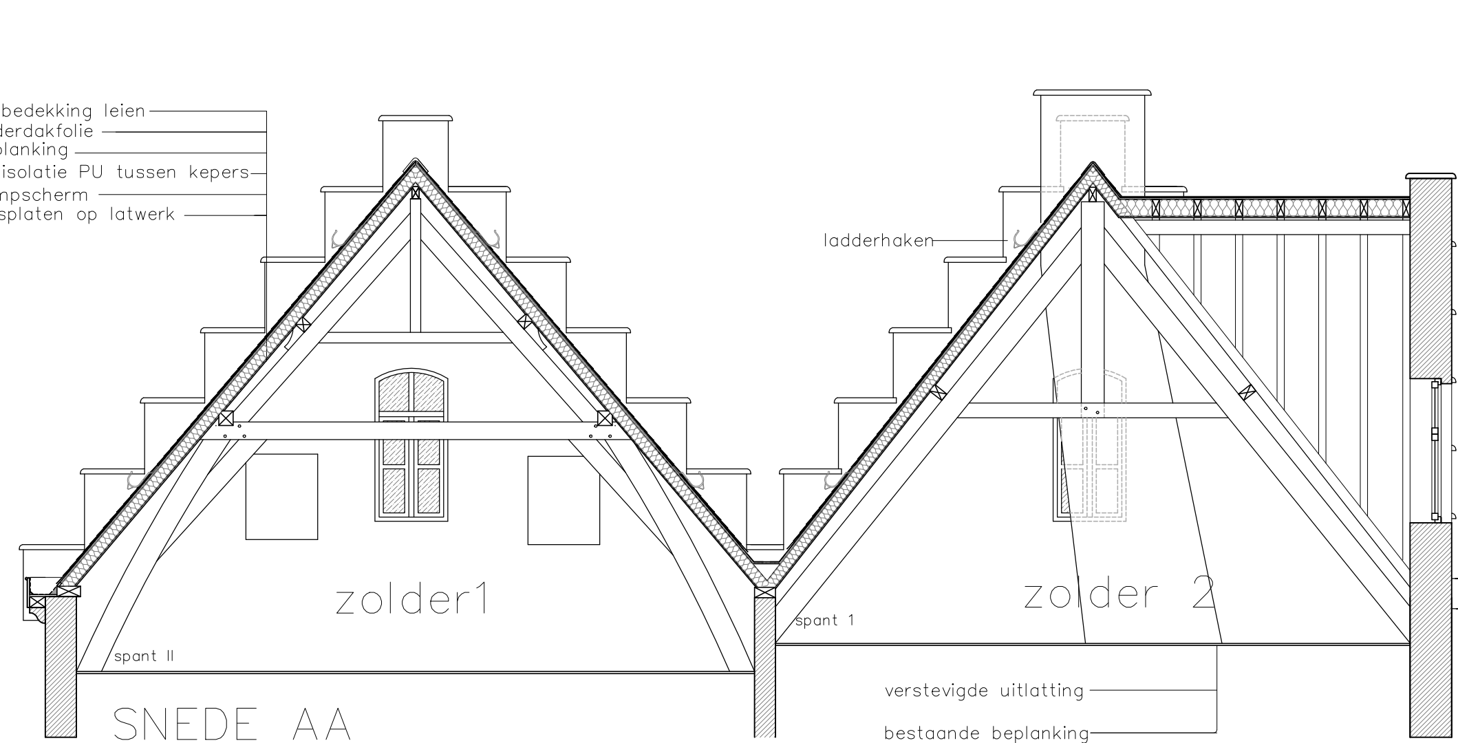
SNEDE AA
