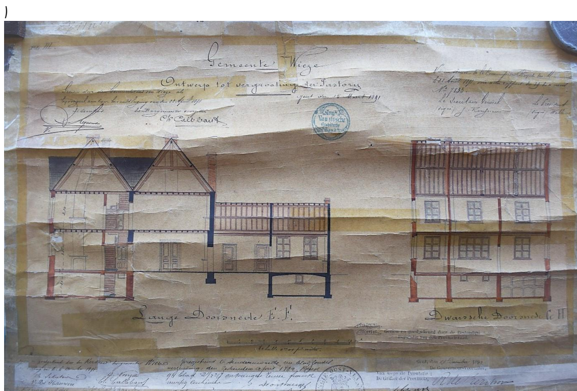
Figuur 12: Plan met doorsneden uit 1891 door August Van Assche (RAG, PAR 399, nr. 41)
