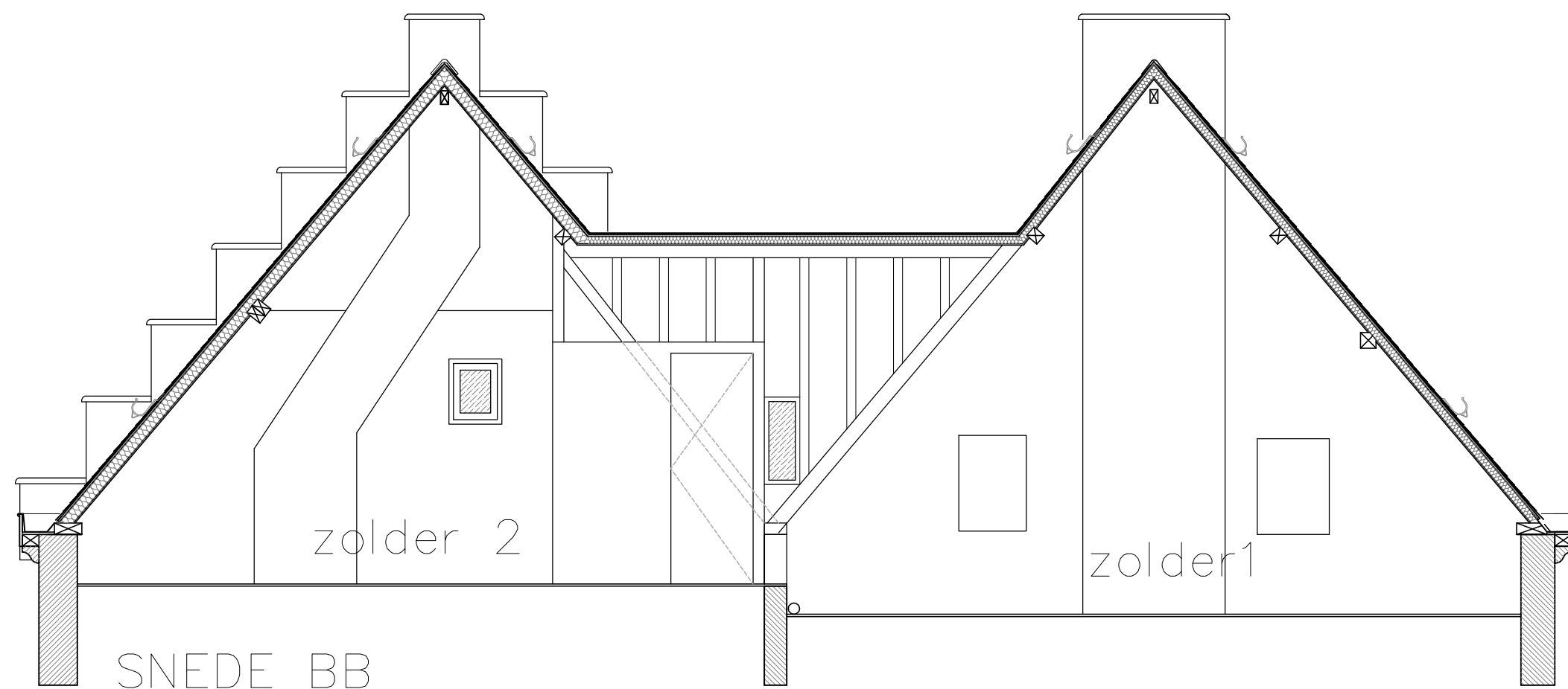
SNEDE BB
