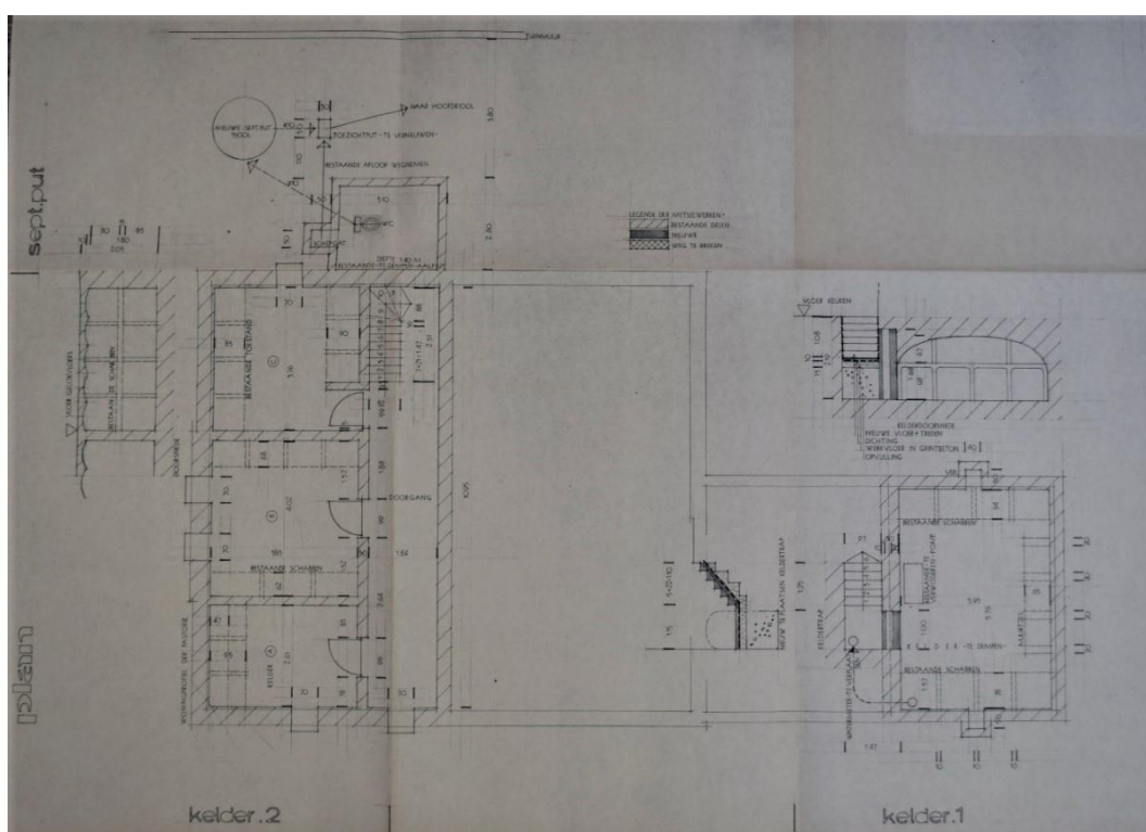
Figuur 33: Grondplan n.a.v. verbouwingswerken in de kelderverdieping (RAG, PAR 399 nr. 47)
