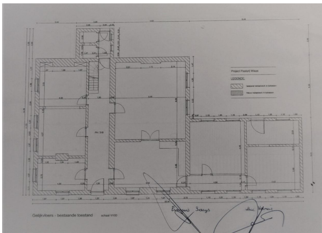
Figuur 39: Gelijkvloerse verdieping bestaande toestand (AOEOVL., beheersdossier pastorie Wieze)
