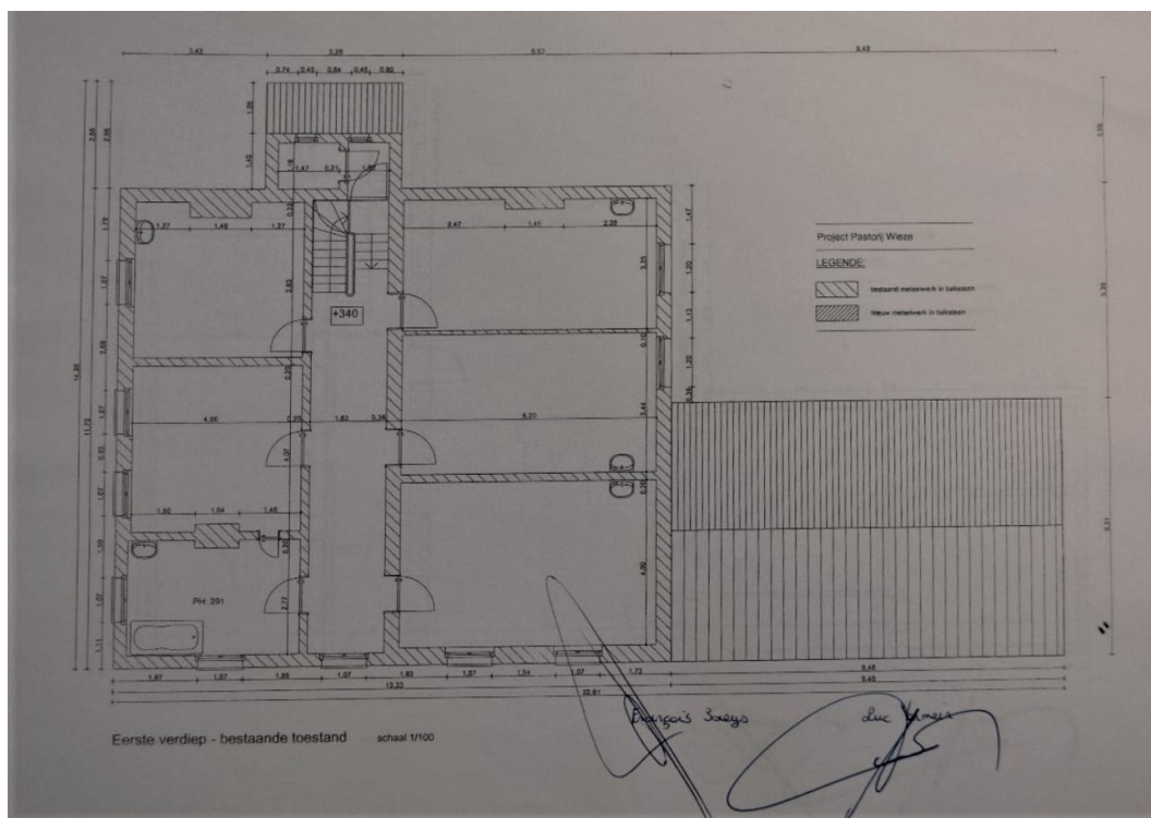
Figuur 40: Eerste verdiep bestaande toestand (AOEOVL., beheersdossier pastorie Wieze)
