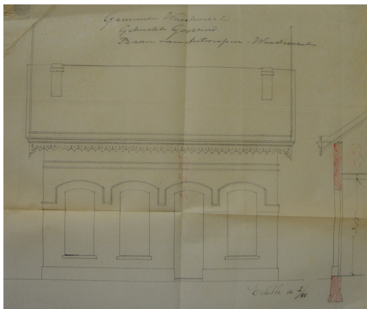
Figuur 6: Gevelplan hovenierswoning, 1880. RAA, Archief van het Departement van de Twee Neten en van de Provincie Antwerpen, Vergunningsaanvragen voor bouwwerken langs rijks- en provinciewegen, nr. 198/45.
