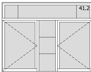
TH B 15 (40.11.2.15) 3-ledig raamgeheel met bovenlicht (230 cm b x 180 cm h) type: inlegraam positie: achter slag beglazing: K 1.0 beslag: recuperatie espagnoletsluiting situering: gelijkvloers - eetkamer aantal: 1
