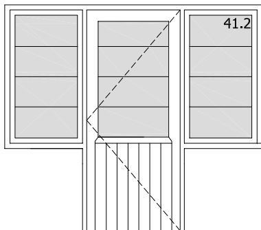
TH B 20 (40.11.2.20) 3-ledig raam- en deurgeheel (248 cm b x 138/217 cm h) type: inlegraam/inlegdeur positie: in slag beglazing: K 1.0 situering: gelijkvloers - keuken aantal: 1
