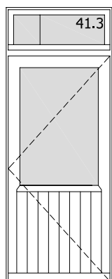
TH B 05 (40.11.2.5) deur geheel met bovenlicht (257 cm b x 100 cm h) type: inlegraam positie: achter slag beglazing: K 1.0 / zonnwerend situering: 1ste verdieping - kamer 1 aantal: 1
