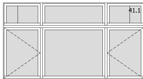
TH A 01 (40.11.1.1) 3-ledig raamgeheel met 3-ledig bovenlicht (311 cm b x 172 cm h) type: inlegraam positie: achter slag beglazing: K 1.0 / zonnwerend / verdund dubbel glas (41.1) situering: gelijkvloers - woonkamer aantal: 1
