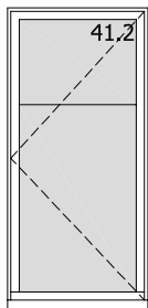
TH B 08 (40.11.2.8) raam (84 cm b x 180 cm h) type: inlegraam positie: achter slag beglazing: K 1.0 / zonnewerend beslag: recuperatie espagnoletsluiting situering: gelijkvloers - eetkamer aantal: 1
