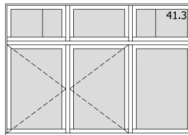
TH B 04 (40.11.2.4) 3-ledig raamgeheel met 3-ledig bovenlicht (242 cm b x 172 cm h) type: Inlegraam positie: achter slag beglazing: K 1.0 / zonnwerend beslag: recuperatie espagnoletsluiting situering: 1ste verdieping - kamer 1 aantal: 1
