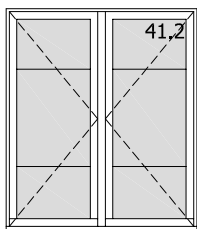
TH B 19 (40.11.2.19) 2-ledig raamgeheel (126 cm b x 149 cm h) type: inlegraam positie: achter slag beglazing: K 1.0 beslag: recuperatie espagnoletsluiting situering: 2de verdieping - kamer 5 aantal: 2
