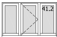
TH B 18 (40.11.2.18) 3-ledig raamgeheel (126 cm b x 81 cm h) type: inlegraam positie: achter slag beglazing: K 1.0 beslag: recuperatie espagnoletsluiting situering: 1ste verdieping - traphal 2 aantal: 2
