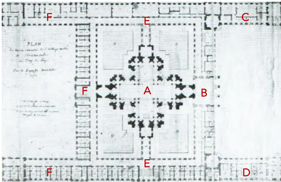
Afbeelding 10: B. Digneffe, Ontwerp voor de abdij van Herkenrode, grondplan, 1773 - Bron: M. Van der Eycken, Herkenrode, abdij en levend monument , Deurne, 2002, p. 108.
