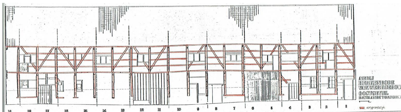
Afbeelding 5: Zusterverblijven, oostgevel - toestand 1981 met aanduiding van de oorspronkelijke balken in rood - Bron: Beerten S., Onderzoek van het vakwerkgebouw van de abdij van Herkenrode , onuitgegeven licentiaatsverhandeling, deel 2, K.U.Leuven, 1981, plan B.
