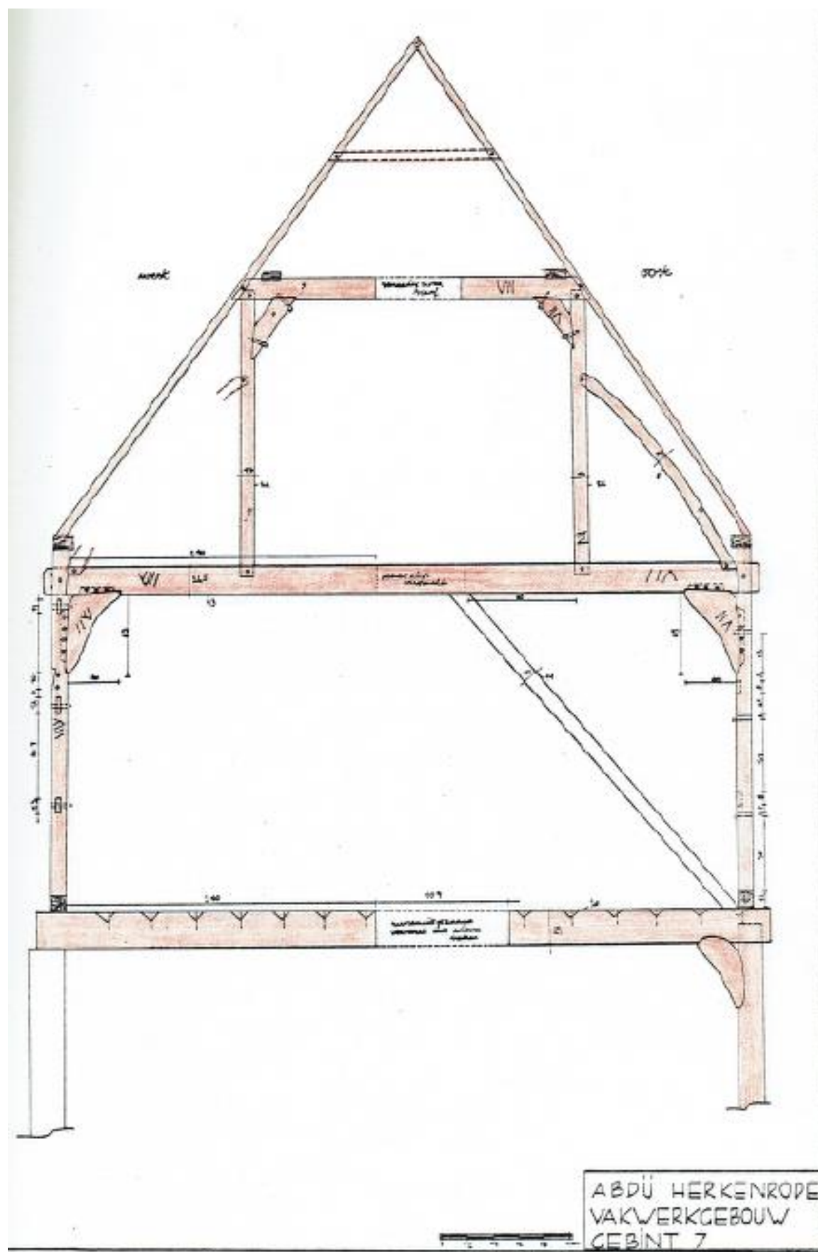
Plan 10: gebint nr. 7, toestand 1981 - Bron: S. Beerten, Onderzoek van het vakwerkgebouw van de Abdij van Herkenrode , onuitgegeven licentiaatsverhandeling, K.U.Leuven, 1981, deel II, opmetingstekening 7
