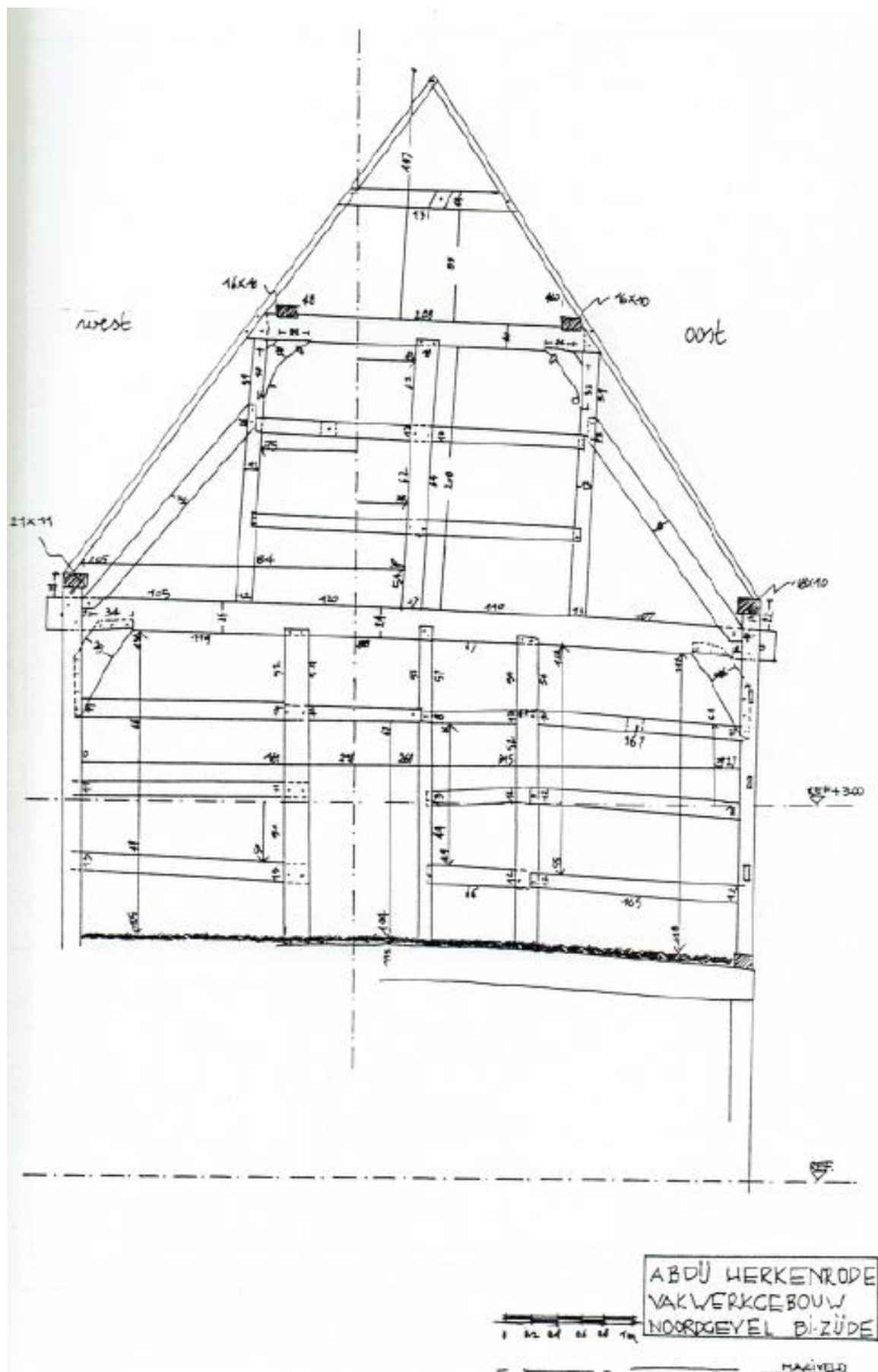
Plan 7: Noordgevel, binnenzijde, toestand 1981 - Bron: S. Beerten, Onderzoek van het vakwerkgebouw van de Abdij van Herkenrode , onuitgegeven licentiaatsverhandeling, K.U.Leuven, 1981, deel II, opmetingstekening 1
