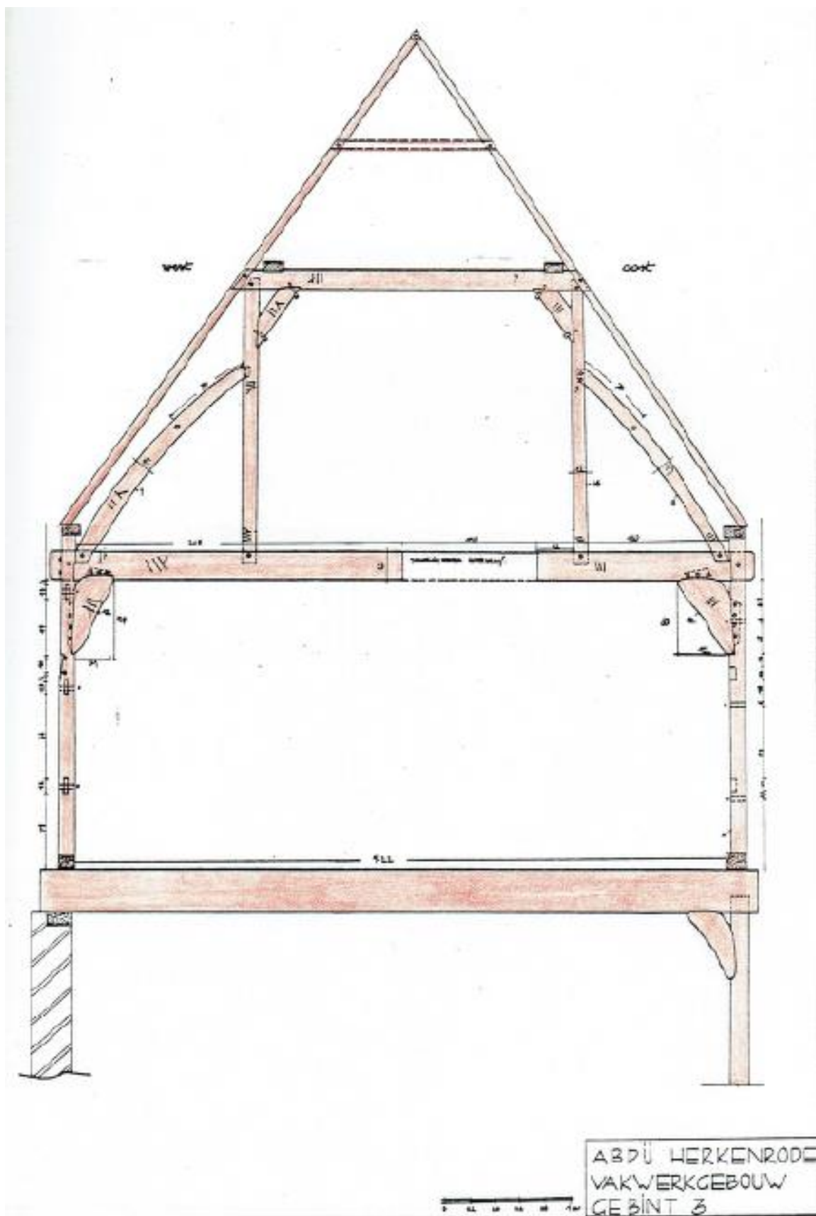
Plan 9: gebint nr. 3, toestand 1981 - Bron: S. Beerten, Onderzoek van het vakwerkgebouw van de Abdij van Herkenrode , onuitgegeven licentiaatsverhandeling, K.U.Leuven, 1981, deel II, opmetingstekening 3
