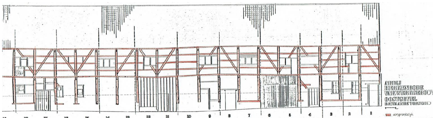
Plan 2: Oostgevel, toestand 1881 - Bron: S. Beerten, Onderzoek van het vakwerkgebouw van de Abdij van Herkenrode , onuitgegeven licentiaatsverhandeling, K.U.Leuven, 1981, deel II, plan B
