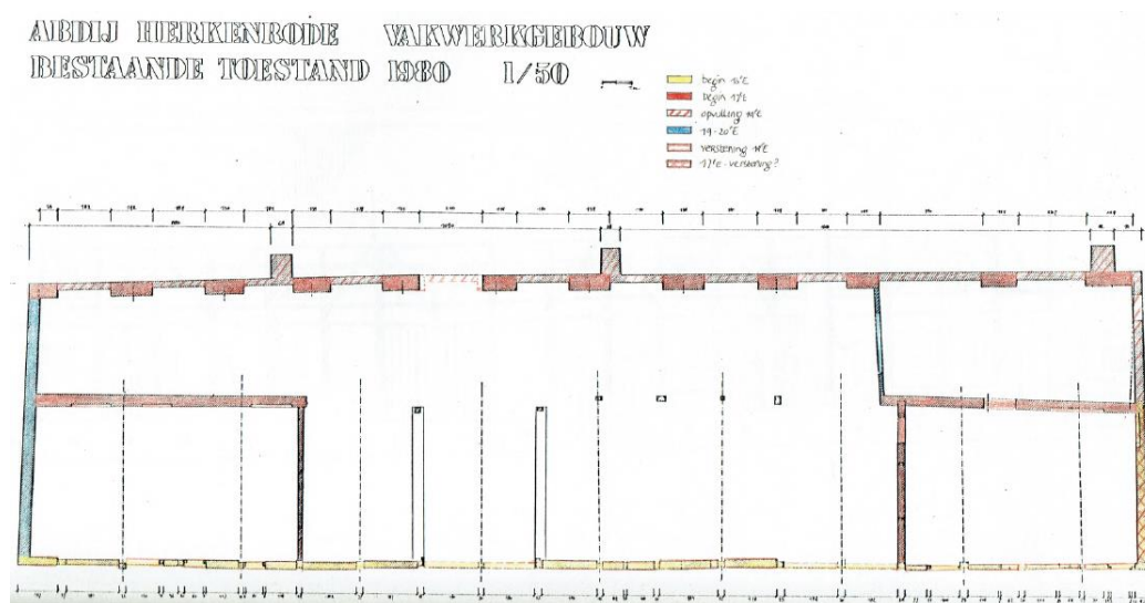
Afbeelding 6: Zusterverblijven, grondplan - Bron: Beerten S., Onderzoek van het vakwerkgebouw van Herkenrode , onuitgegeven licentiaatsverhandeling, K.U. Leuven, deel II, plan A.
