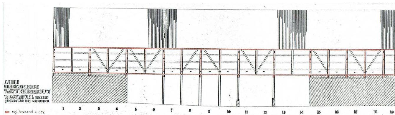
Plan 5: Oostgevel, binnenzijde, toestand 1981 - Bron: S. Beerten, Onderzoek van het vakwerkgebouw van de Abdij van Herkenrode , onuitgegeven licentiaatsverhandeling, K.U.Leuven, 1981, deel II, plan E
