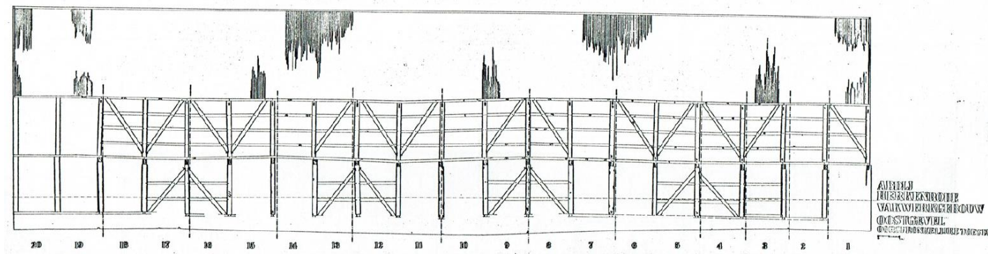
Plan 3: Oostgevel, vermoedelijke oorspronkelijke opstand - Bron: S. Beerten, Onderzoek van het vakwerkgebouw van de Abdij van Herkenrode , onuitgegeven licentiaatsverhandeling, K.U.Leuven, 1981, deel II, plan C
