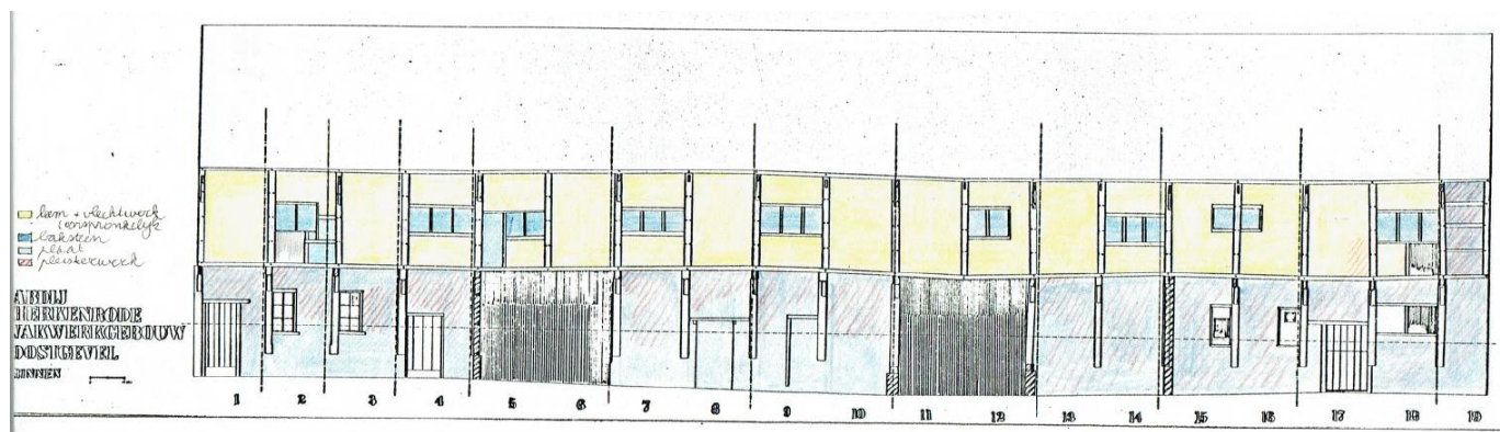
Plan 4: Oostgevel, binnenzijde, toestand 1981 - Bron: S. Beerten, Onderzoek van het vakwerkgebouw van de Abdij van Herkenrode , onuitgegeven licentiaatsverhandeling, K.U.Leuven, 1981, deel II, plan D
