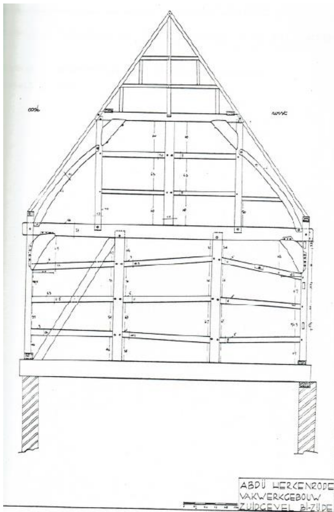
Plan 8: Zuidgevel, binnenzijde, toestand 1981 - Bron: S. Beerten, Onderzoek van het vakwerkgebouw van de Abdij van Herkenrode , onuitgegeven licentiaatsverhandeling, K.U.Leuven, 1981, deel II, opmetingstekening 21
