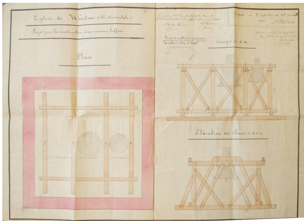
Figuur 19 : Ontwerp van Frans De Flander uit 1888 voor een nieuwe klokkenstoel (Stadsarchief Ieper).
