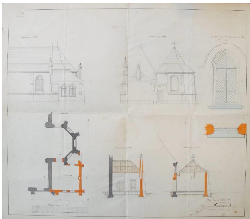
Figuur 18 : Plan van architect G. Lernoould voor een nieuwe sacristie in 1863 (Stadsarchief Ieper)
