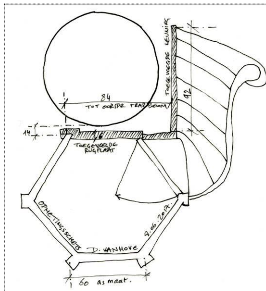
Figuur 117 : opmetingsschets van de kuip van de preekstoel (D. Vanhove 8.06.2017)
