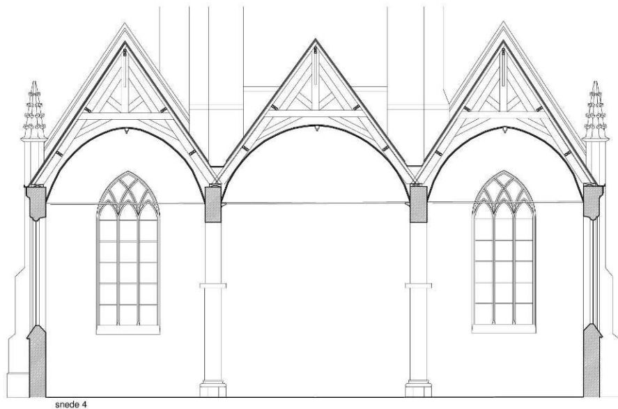
Figuur 174 : Tekening doorsnede over de zadeldaken (Dries Vanhove architectenbureau).
