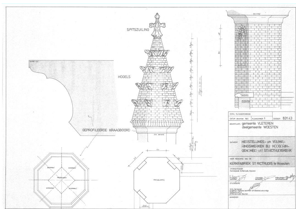
Figuur 54: Detailplan flanketorentje van vieringstoren door Arch. Willy De vriendt, gedateerd 1983 (kerkarchief Woesten).
