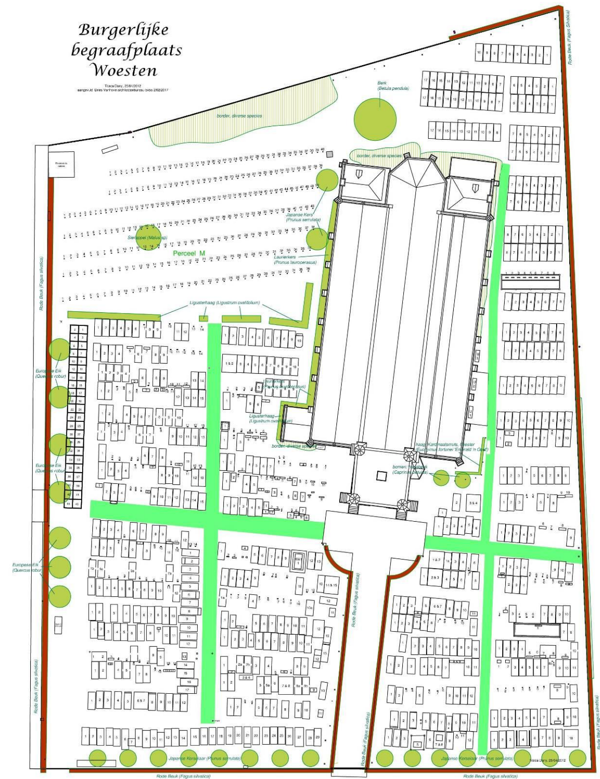
Figuur 186 : Aanleg en groenaanleg kerkhof Woesten (opmetingsplan Dany Titeca 2012, opgewerkt Dries Vanhove architectenbureau bvba) (zie ook A3 versie in bijlage).
