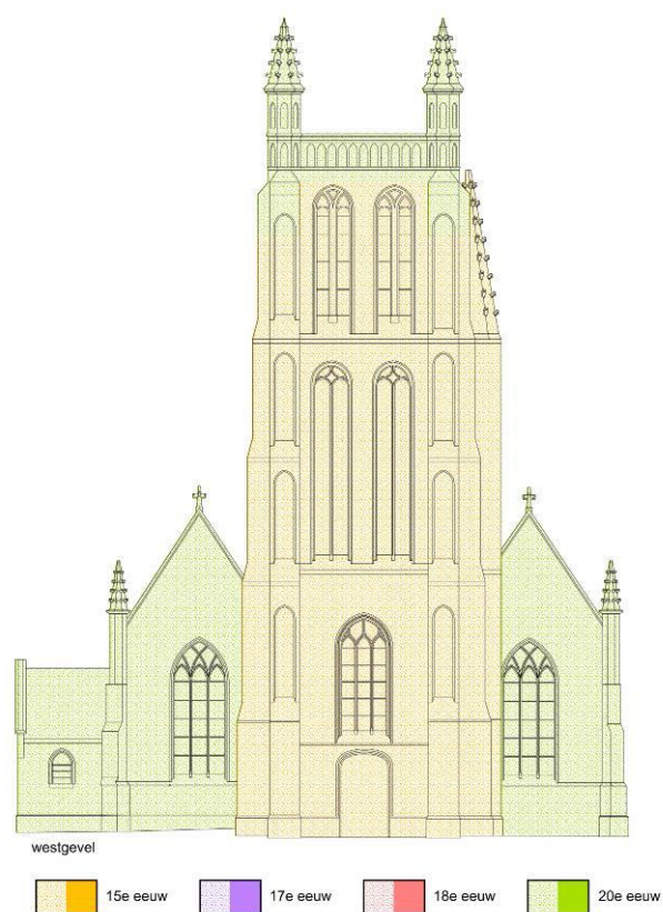
Figuur 6 : Gevelplan van de westgevel, met aanduiding van de bouwperiodes.
