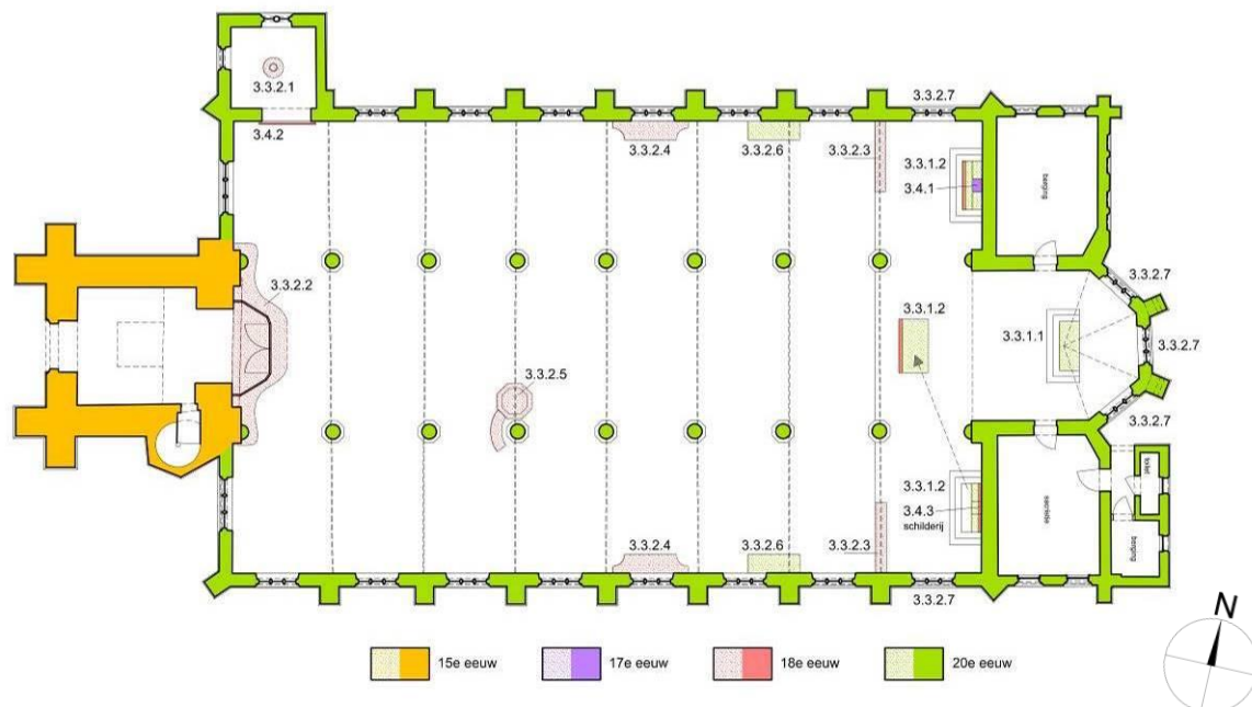
Figuur 5 : Grondplan van de Sint-Rictrudiskerk met bouwperiodes. De nummering van de erfgoedelementen verwijst naar de nummering in deel 3 van het beheersplan.
