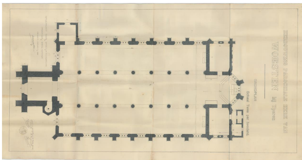
Figuur 38: Grondplan - architecten J. en W. Vercoutere, oktober 1920 (Kerkarchief Woesten).
