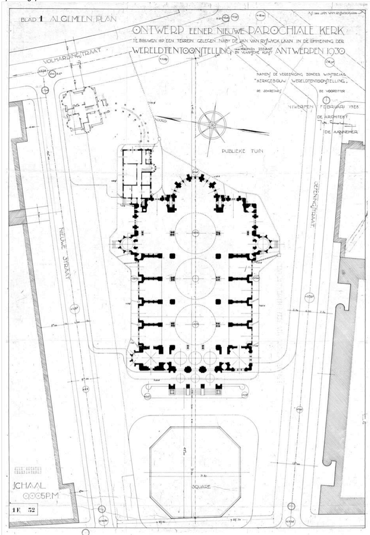
Figuur 25: Inplantingsplan
