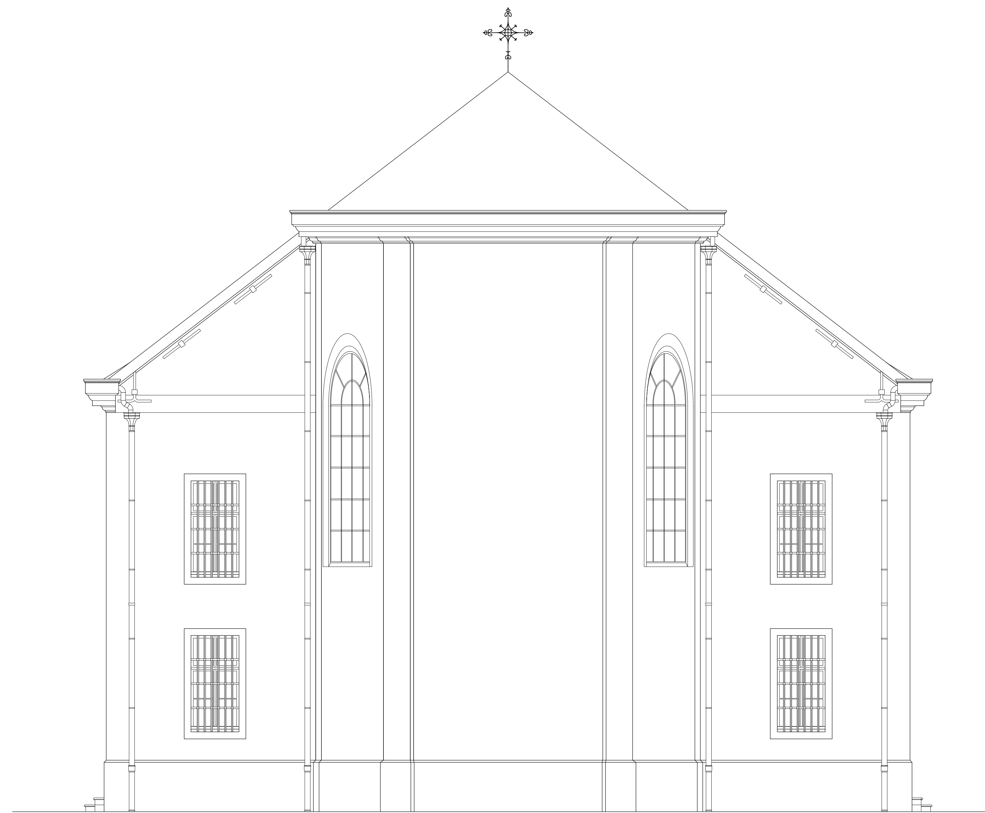
GEVEL OOST
