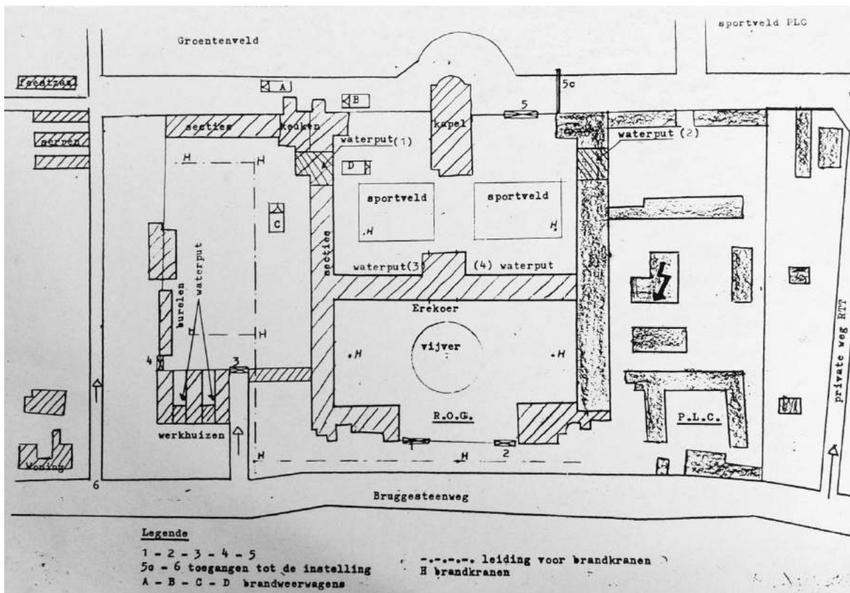
Afbeelding 2-74: Plan van de gebouwen van het ROG en PLC op grondgebied Ruiselede anno 1984 (naar aanleiding van een brandveiligheidsoefening). Bron: RAB, Archief ROG Ruiselede en Beernem (2000), nr. 444.
