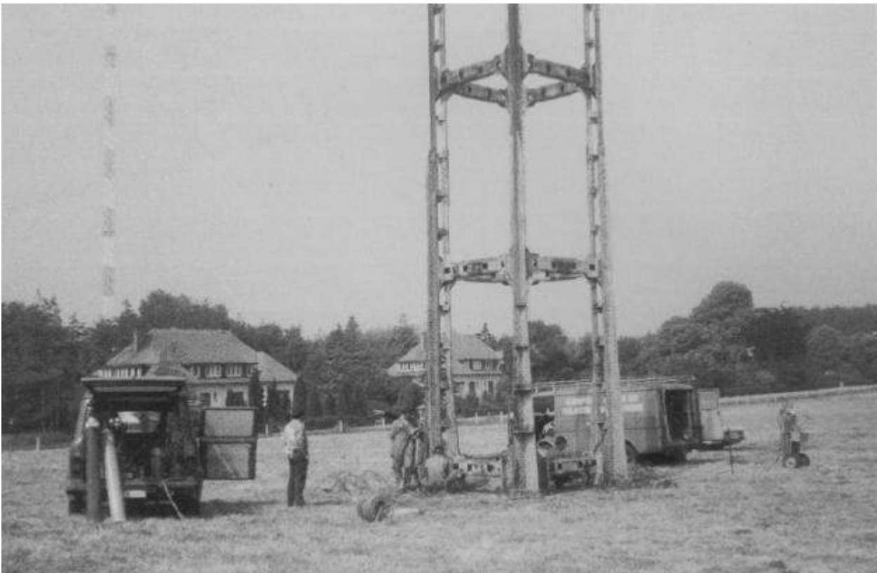
Afbeelding 2-66: Sloop van het resterende geraamte van pyloon nr. 6, op 23 juli 1979, met op de achtergrond de personeelswoningen van de RMD (SCRE) gebouwd in 1954. Bron: Arnoys & Ghyselbrecht, Geschiedenis van het Zendcentrum SCRE te Ruiselede/Wingene en de dienst Belradio , p. 139.
