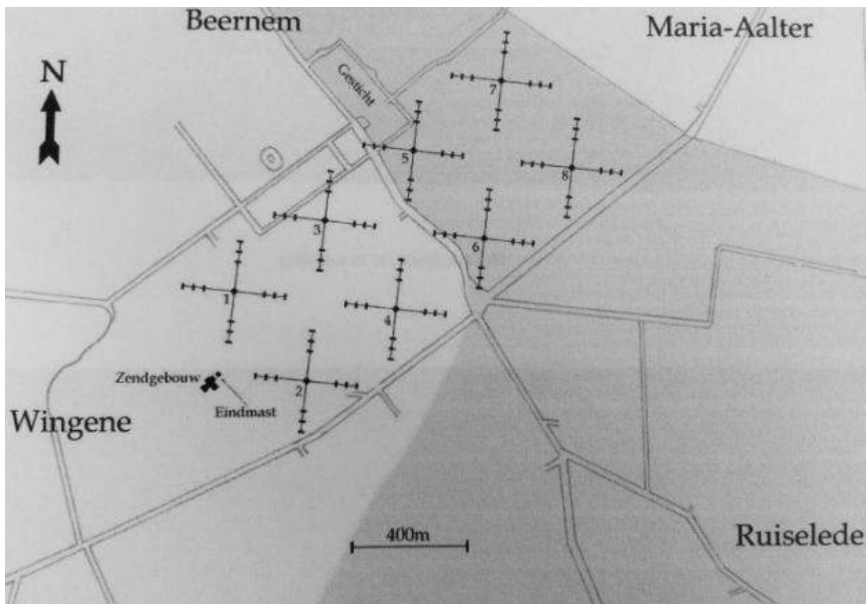
Afbeelding 2-59: Plan gemaakt door Ghyselbrecht met inplanting en nummering van de zendtorens. Bron: Arnoys & Ghyselbrecht, Geschiedenis van het Zendcentrum SCRE te Ruislede/Wingene en de dienst Belradio , p. 47.
