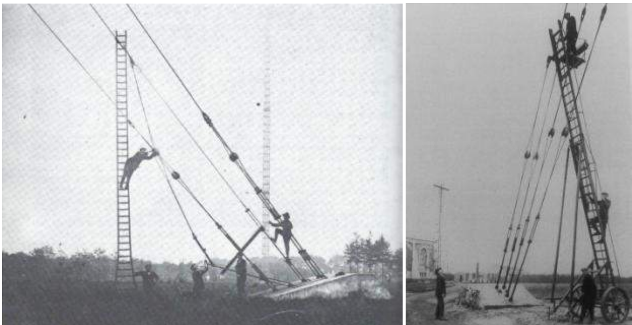
Afbeelding 2-60: Het aanspannen van de kabels van de torens, verbonden aan het betonnen ankervoetstuk. Foto links van ingenieur Van Lierde. Bron: Baelde, “De Torens van Ruislede” , p. 118. Bron foto
