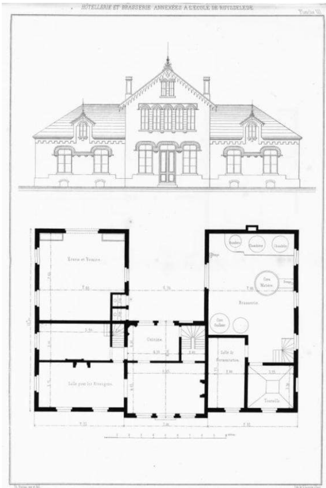
Afbeelding 2-112: Voorgevel en grondplan van de hotellerie en de brouwerij bij het ROG uit 1855-1856, met de originele "corniche". Bron: Ducpétiaux, Exposé de la Situation des écoles de réforme de Ruysselsede, de Wyngheene et de Beernem , planche III.
