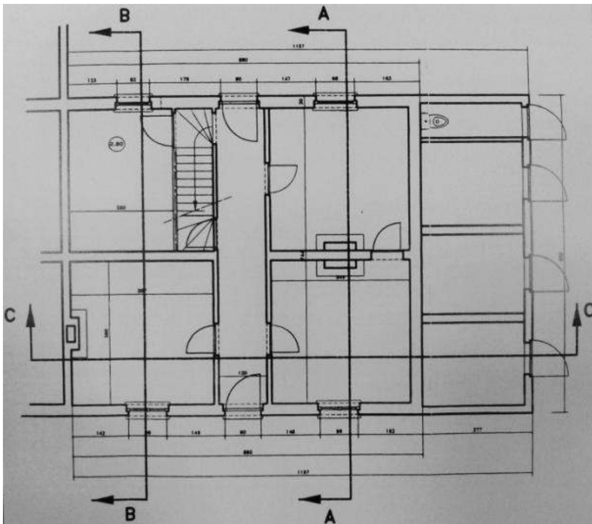
Afbeelding 2-136:: Voorgevel en plattegrond van het gelijkvloers van één van de dubbelwoningen die als surveillantenhuisjes ter beschikking gesteld werden van het ROG-personeel. Huidig adres: palend aan de Boskapeldreef, Sint-Pietersveld nr. 16, de hoekwoning naast het O.C. Wingene. Bron: Vercruysse, "Ons familieleven in Sint-Pietersveld en Oedelem (1933-1945)", pp. 175-176).
