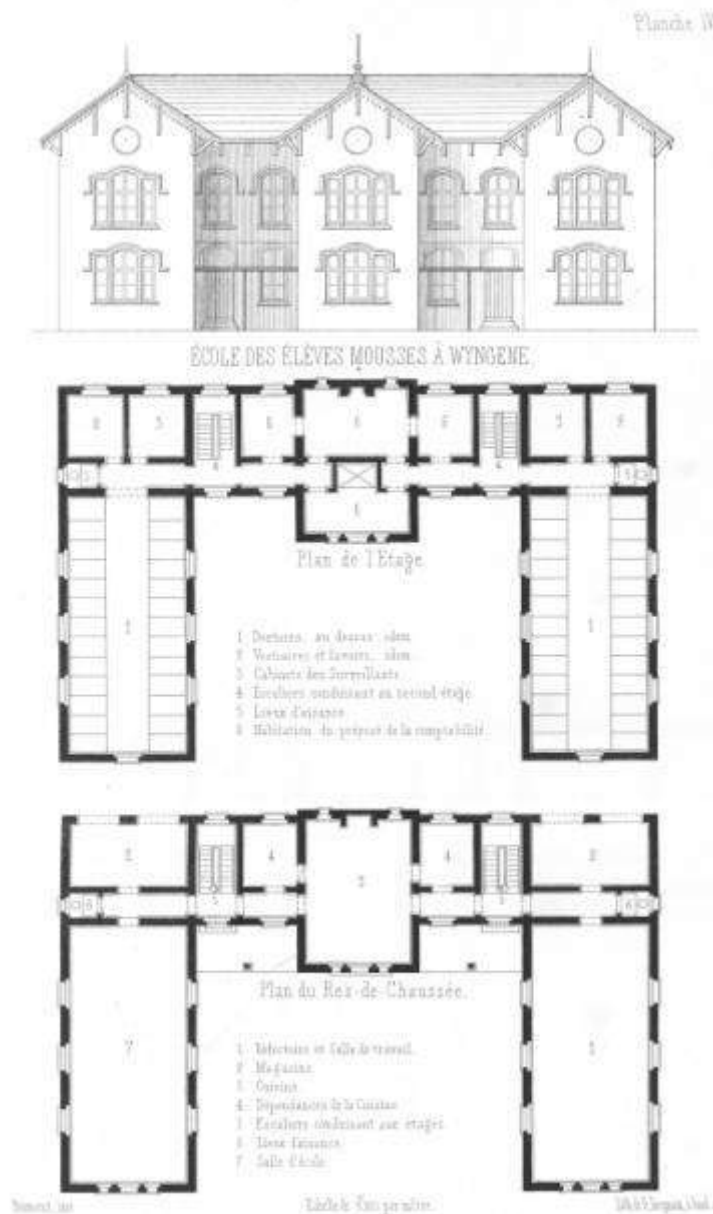
Afbeelding 2-120: Oorspronkelijk gevelaanzicht en grondplannen voor de “ école des mousses ” door architect Dumont. Oorspronkelijke E-vormige gebouw. De bedaking werd uiteindelijk heel wat soberder gehouden. Gepubliceerd in 1861. Bron: Ducpétiaux, Exposé de la Situation des écoles de réforme de Ruysselede, de Wyngene et de Beernem , planche IV.
