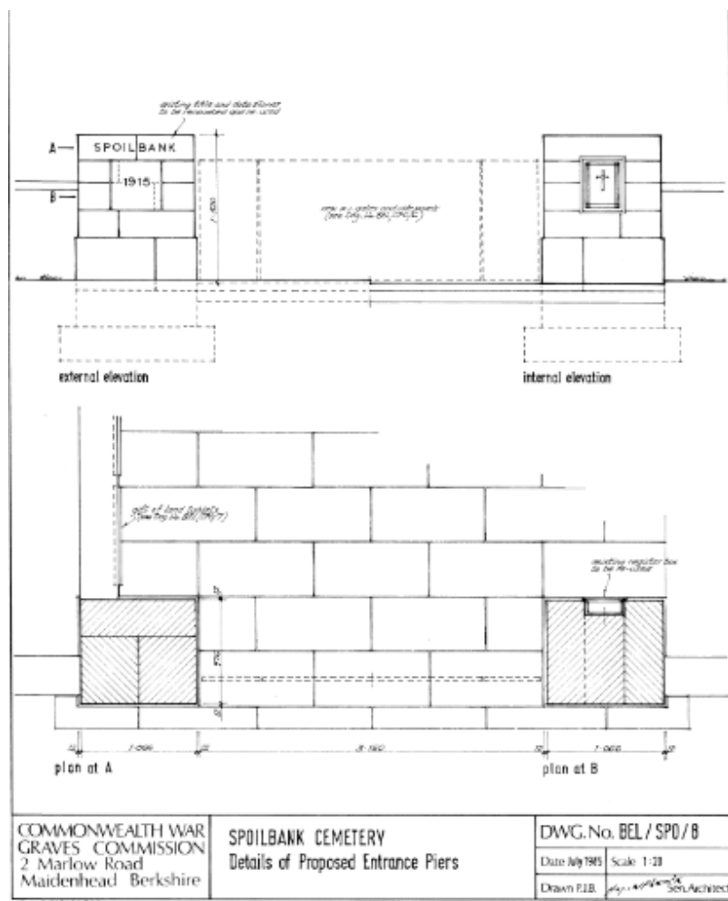
Figuur 5. Plan met nieuwe ingangselement (1985)
