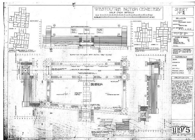
Figuur 3. Westoutre British Cemetery | 'Details', gedateerd 20 juli 1922
