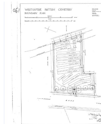
Figuur 1. Westoutre British Cemetery | 'Boundary Plan', gedateerd 31 augustus 1920 2
