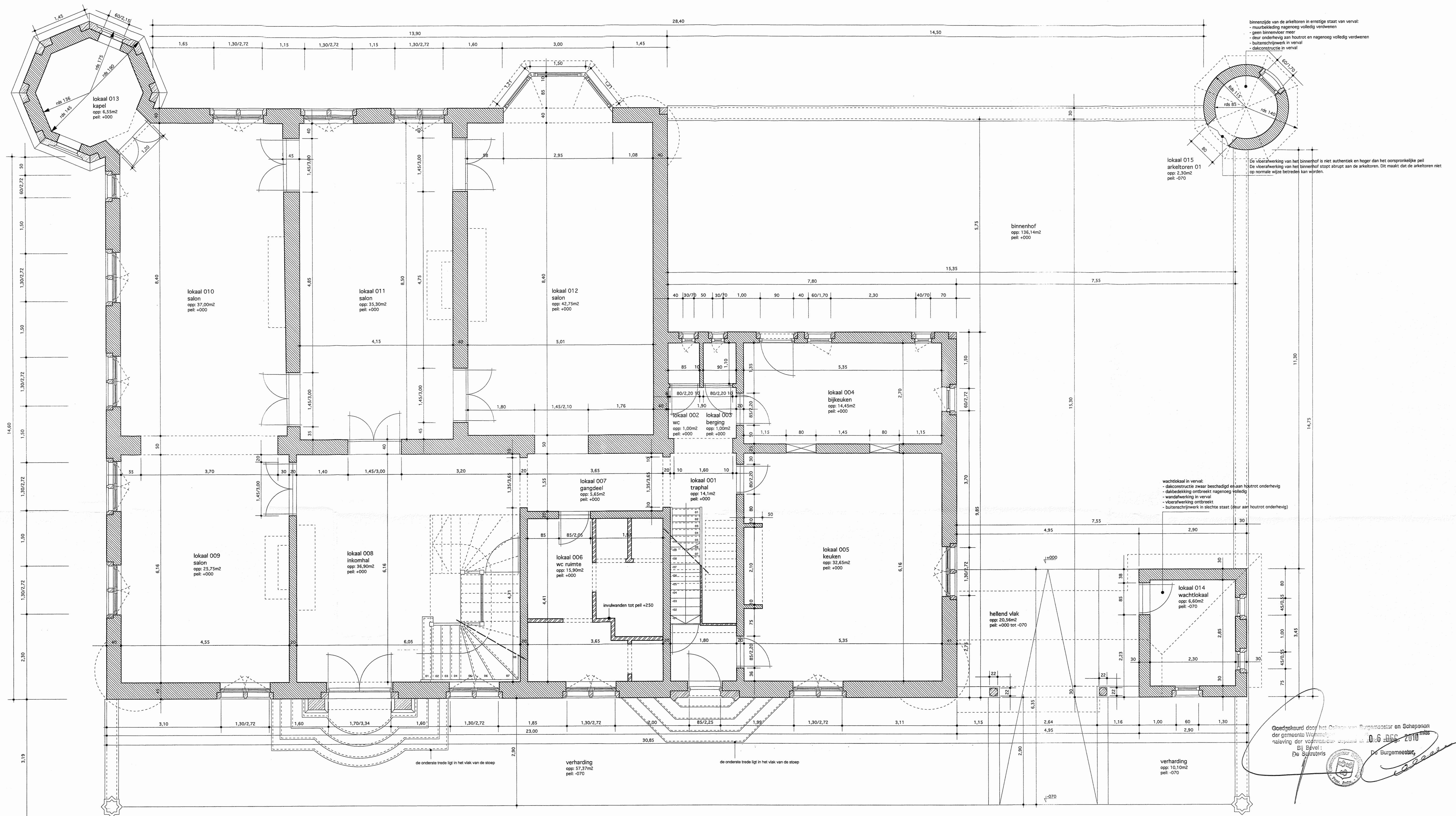
GELIJKVLOERS - OPMETINGSPLAN schaal 1/50
