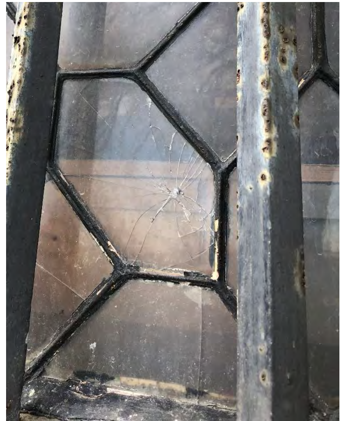
Foto's boven: glasramen van de sacristie met meer figuratieve veelhoekige vormen. Enkel glas zit met fijne mastiekrand vast in een metalen frame en is eerder zeldzaam.
