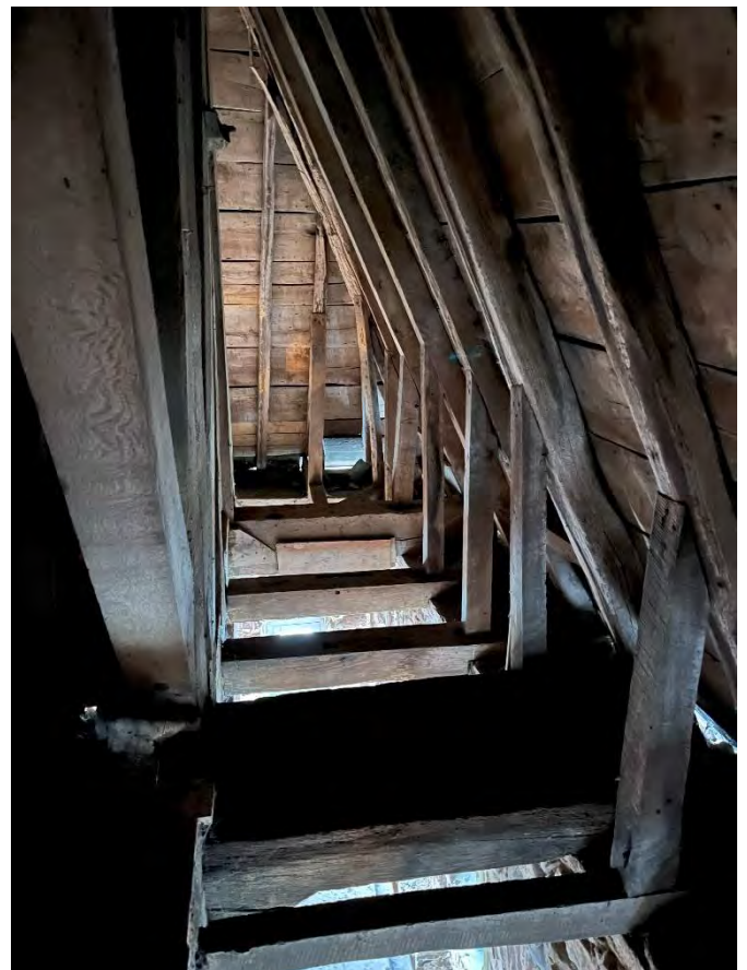
Nivo onder de klokkenstoel met diagonale steunstructuur voor bovenstaande klokkenstoel. Ontbrekende planken op kepers aan buitenzijde om inspectie mogelijk te maken.
