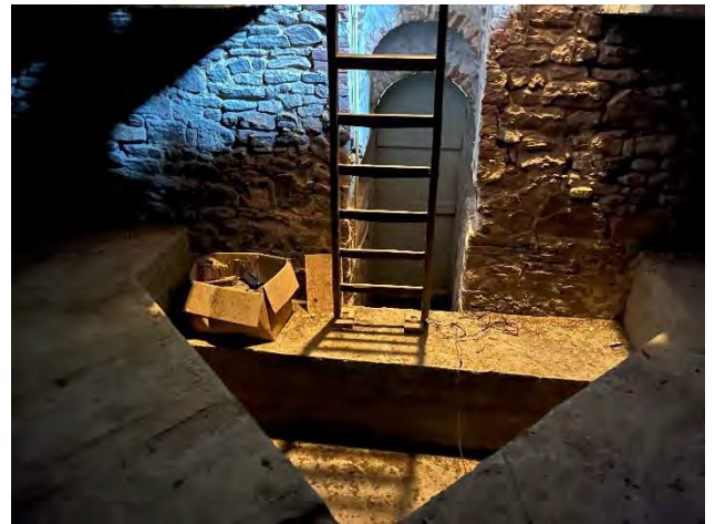
Toegangsdeur oostzijde met houten ladder naar bovenliggend nivo.
