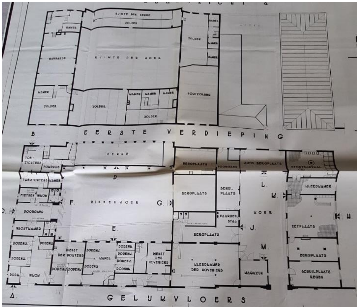
Figuur 26: een plan uit de jaren 1960 (architect Ferdinand Peeters) geeft ons een beter beeld van de ruimten die uiteindelijk ontwikkeld werden, zoals de dodencellen, ruimte voor dokters, enz. (bron: archief dienst begraafplaatsen - kasteel Schoonselhof)
