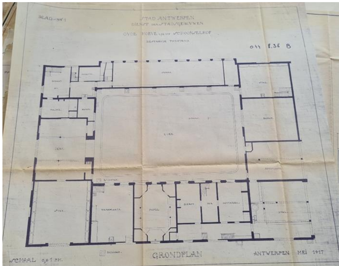
Figuur 25: plan d.d. mei 1917 met eerste ontwerp voor de inrichting van de neerhoeve. In dit ontwerp is er een kapel, naast tal van ruimten voor hoveniers en stelplaatsen. (bron: archief dienst begraafplaatsen - kasteel Schoonselhof)
