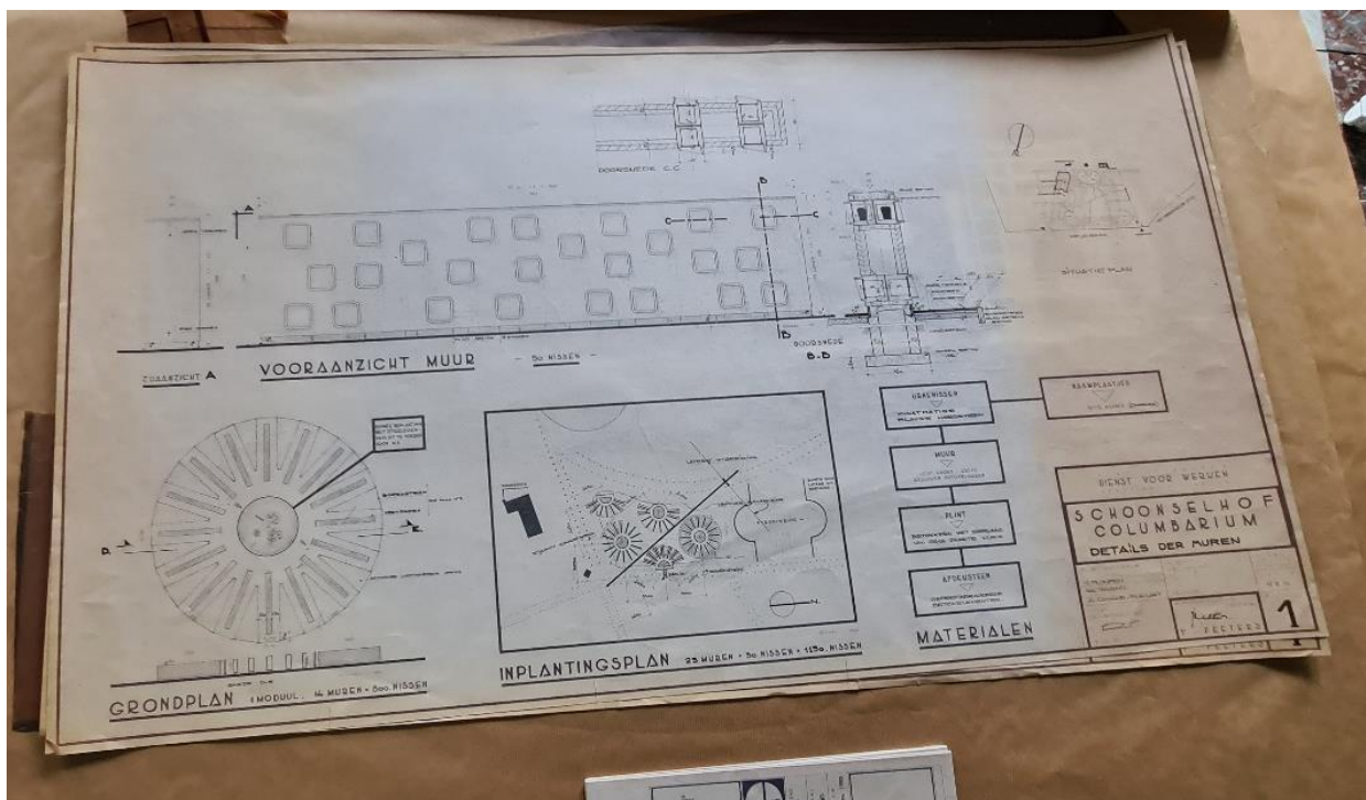
Figuur 2: grondplan en inplantingsplan voor het columbarium (d.d. 12/02/1974) (archief kasteel Schoonselhof)
