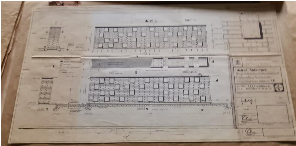
Figuur 8: ontwerp voor uitbreiding bestaande columbariumnissen (nr. IV), december 1993, (architecten: J. De Bruyne, M. Dierckxsens, Taeymans)
