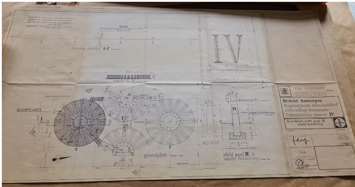
Figuur 9: ontwerp (grondplan) anno 1993 (deel van plan 'uitbreiding bestaande columbariumnissen nr. IV'), december 1993, (architecten: J. De Bruyne, M. Dierckxsens, Taeymans)
