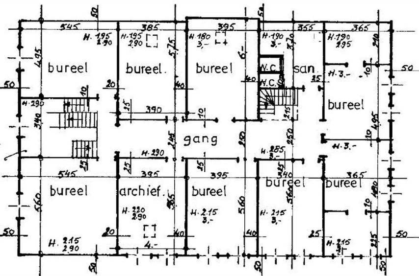
Plantekeningen Hotel Schaetzen (d.d. 12/01/1982), detail tweede etage
