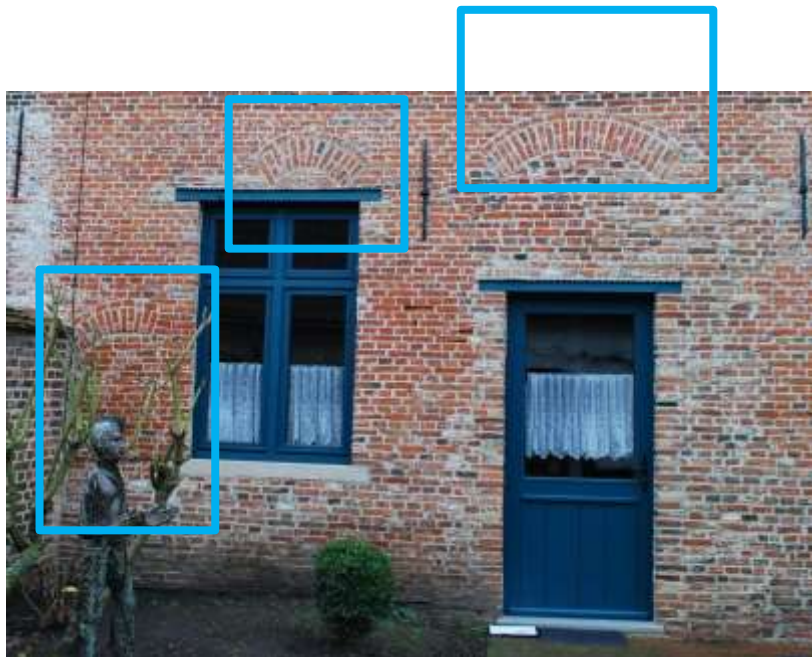
Foto 72 Bouwsporen aanpassingen achtergevel
