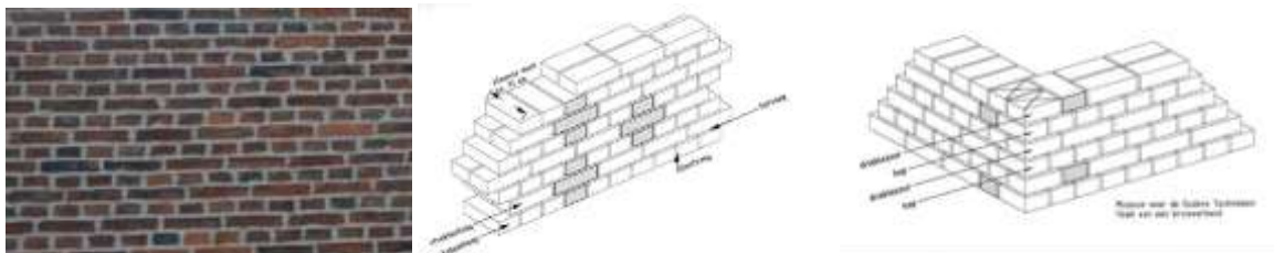
Foto 80 Metselwerkverband: kruisverband (Bron Museum voor Oudere Techniek)
