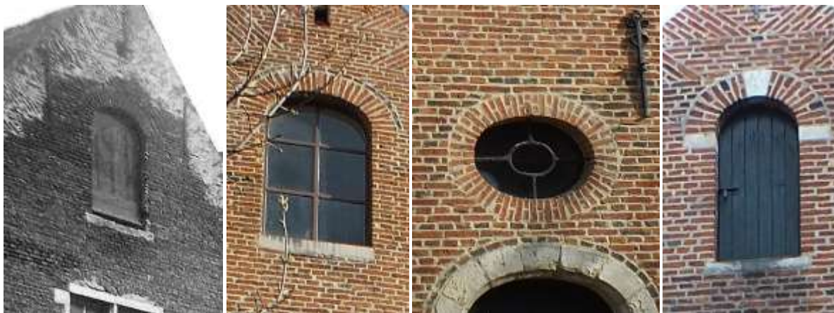
Foto 111 Voorbeelden van raamopeningen in baksteen.
