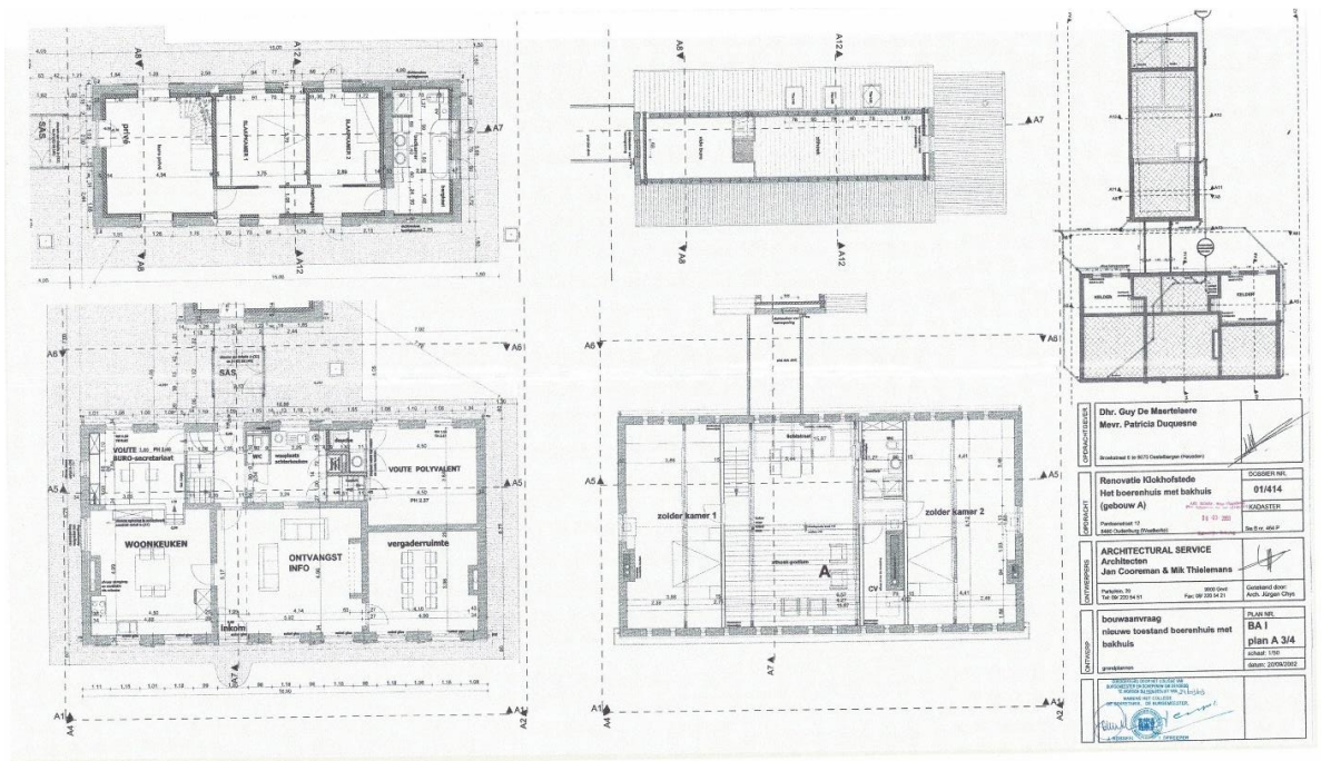
Jan Cooreman & Mik Thielemans, opmetingsplan van het bakhuis, geplande toestand 20/09/2002 in opdracht van Guy De Maertelaere en Patricia Dusuesne.
