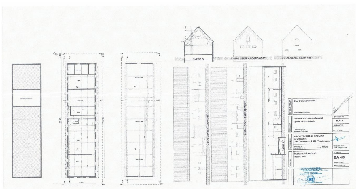
Jan Cooreman & Mik Thielemans, opmetingsplan van de schuur, bestaande toestand en plan voor inbrengen van een vakantieverblijf, 18/03/2002 in opdracht van Guy De Maertelaere.
