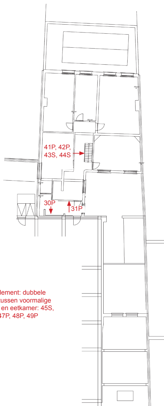
Plan eerste verdieping woning (© Jan Boens)
