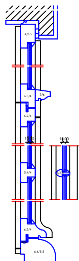
verticale doorsnede 1:10
