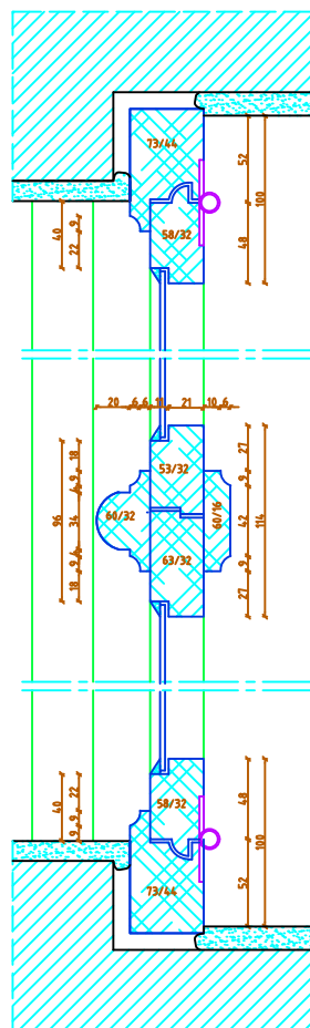
Horizontale doorsnede, opendraaiend
