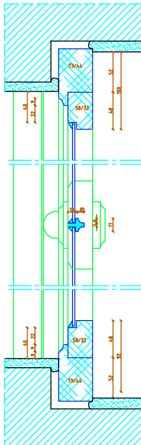
Horizontale doorsnede, bovenlicht
