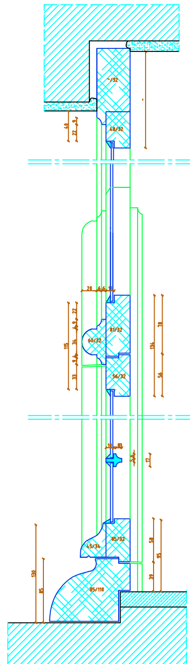
Verticale doorsnede
