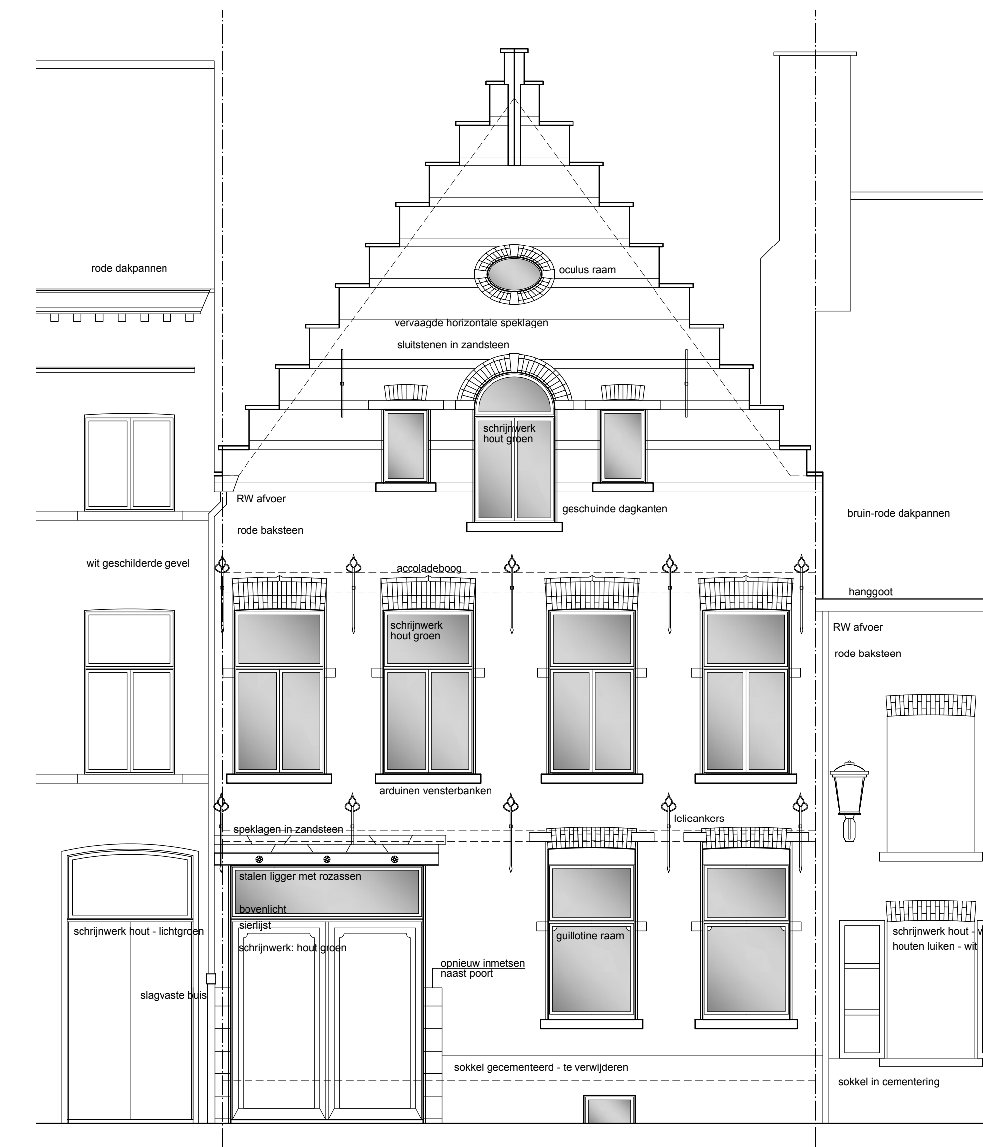
VOORGEVEL
