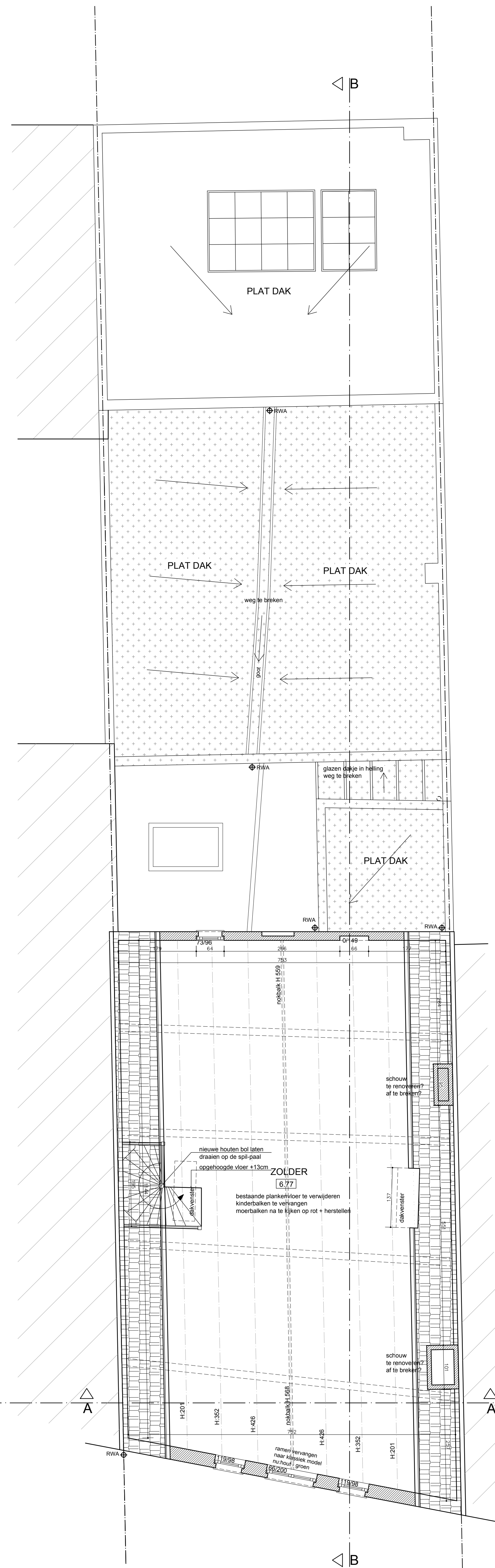
ZOLDER schaal 1/50
