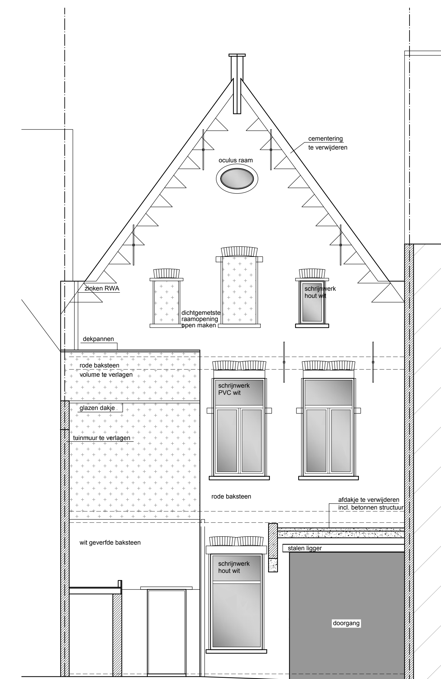
ACHTERGEVEL
