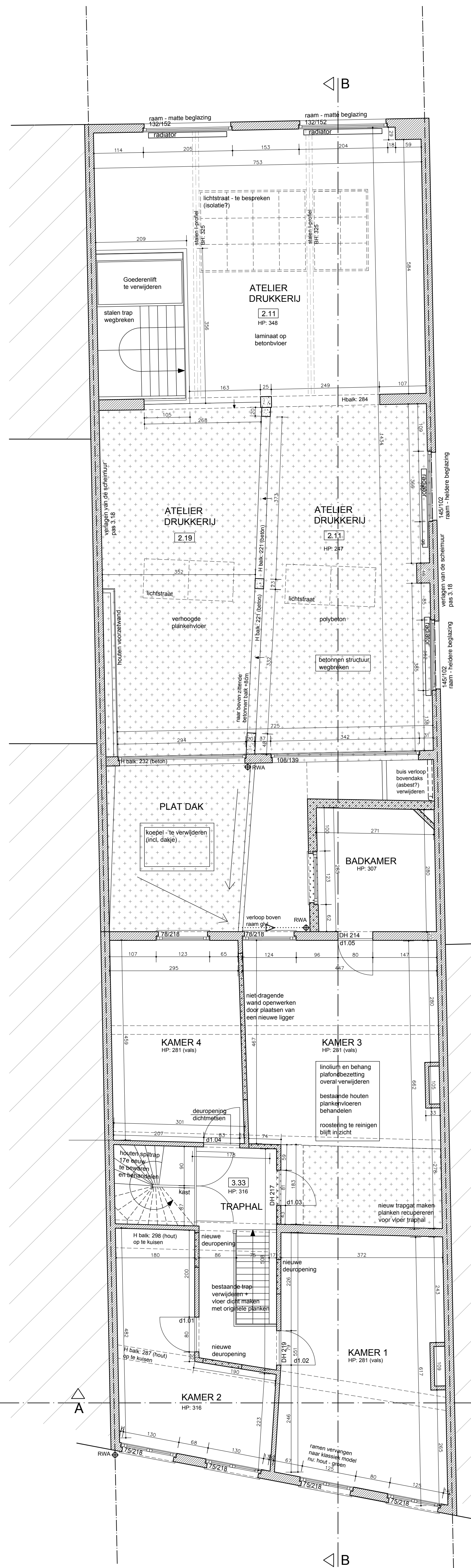
NIVEAU +1 schaal 1/50
