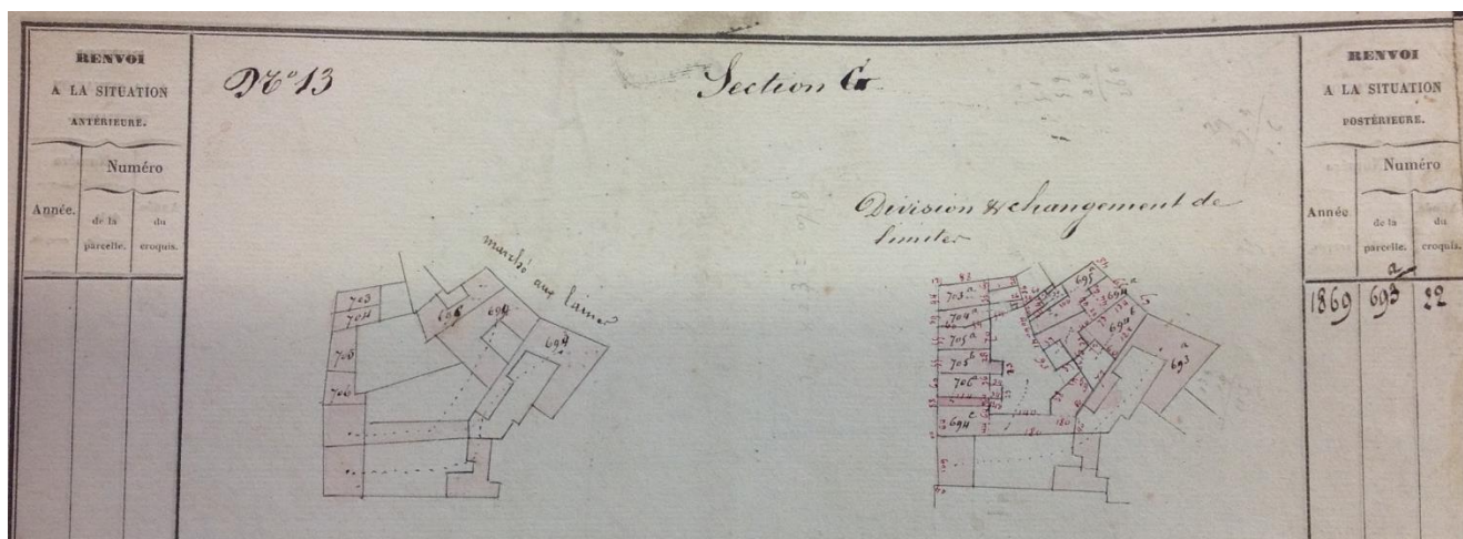
Afb. 2. Tienen, Wolmarkt 15-17: mutatieschets 13, 1858 (Bron: Algemene Administratie van de Patrimoniumdocumentate/opmetingen en waarderingen, Kadaster Leuven, Tienen, 3 de afdeling, Sectie G)
