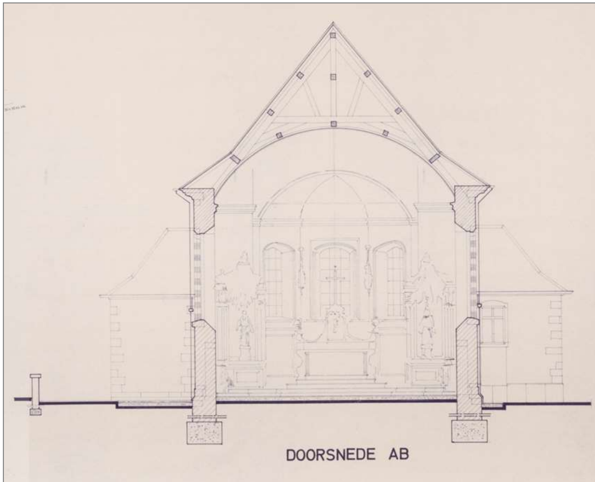
Figuur 6. Doorsnede van de St-Agustinuskerk van Beert. (Architect Victor Soens 1959-1960)
