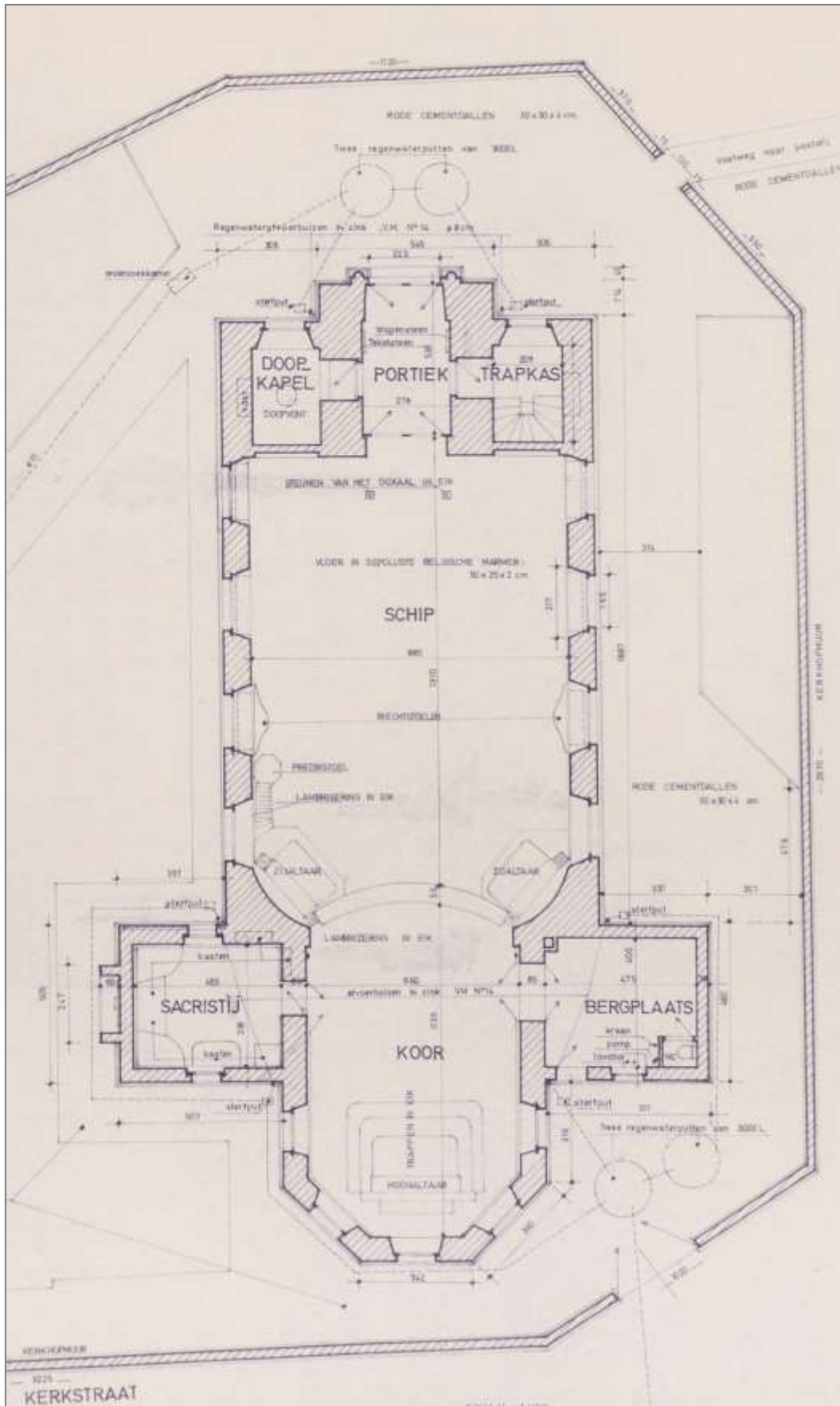
Figuur 3. Grondplan van de St-Augustinuskerk van Beert. (Architect Victor Soens 1959-1960)
