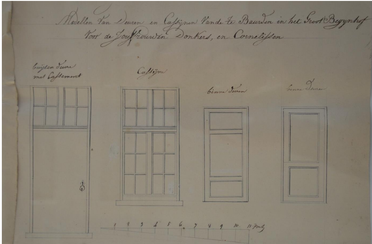
Ontwerptekening voor het buiten- en binnenschrijnwerk van begijnenhuis d'Arke van Noë (Zwarte katstraat 6-8), daterend van 1827 (Bron: OCMW-Archief Gent, BG 11/8).
