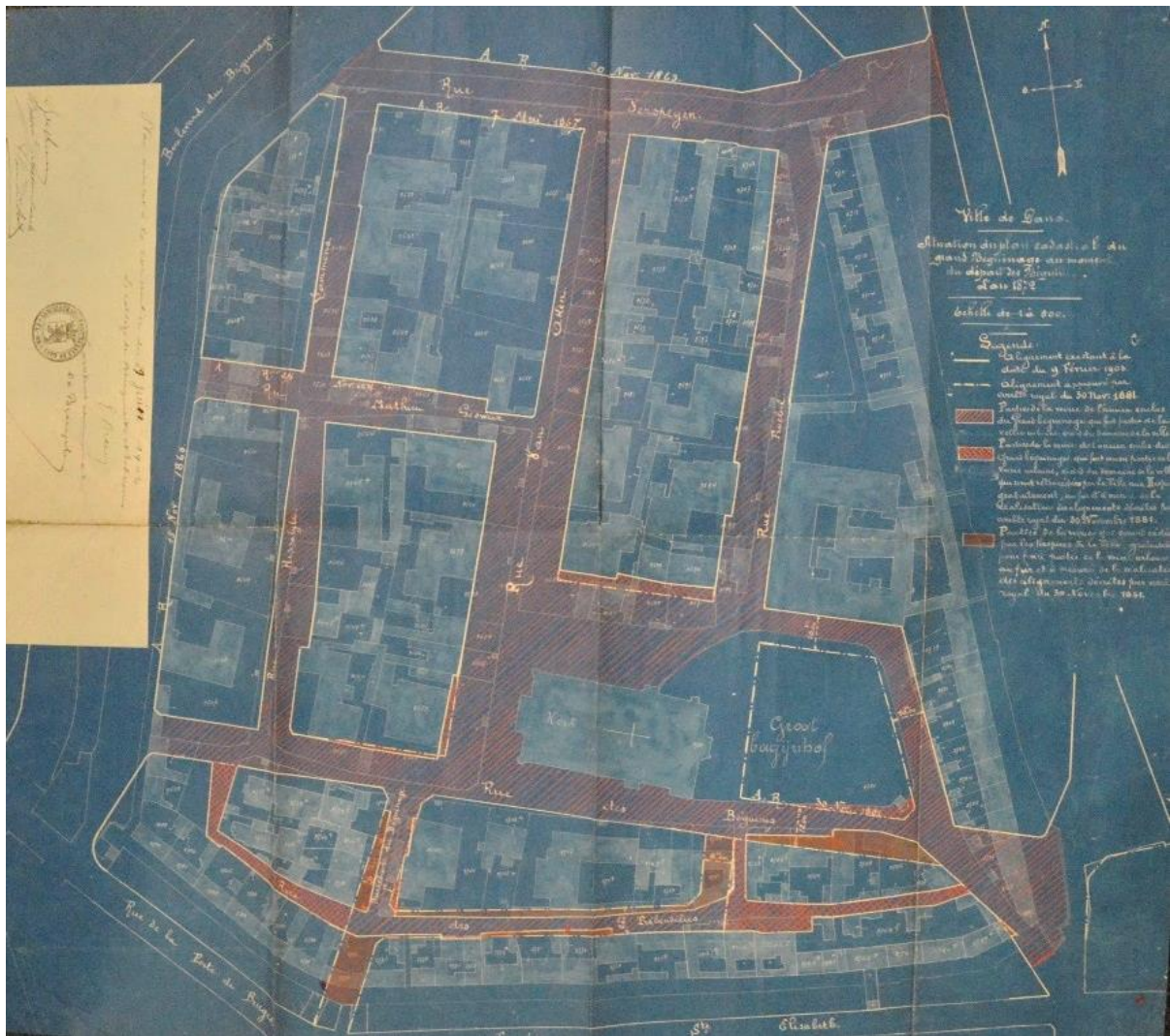
Afb. 9 - Kadastraal plan van 1872, met aanduiding van de rooilijnen in 1903 (volle lijn), met de nog voorziene (niet uitgevoerde) werken, volgens het rooilijnplan van 1881 (stippellijn), waaronder het verlengen van de Zwartekatstraat naar Brugsepoortstraat en de sloop van de huizen ten zuiden van de dries om deze straat volledig te kunnen rechtekken.
