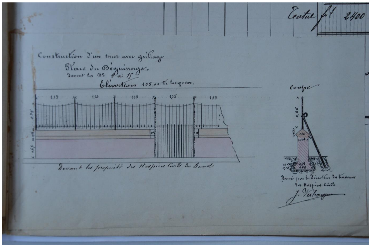
Afb. 18. Ontwerptekening uit 1901 voor de te vernieuwen omheiningsmuurtjes langs de zuidzijde van de kerk (huidige Begijnhofdries) (Bron: Archief Gent, Archief OCMW Gent, BG11 Begijnhoven, 63).
