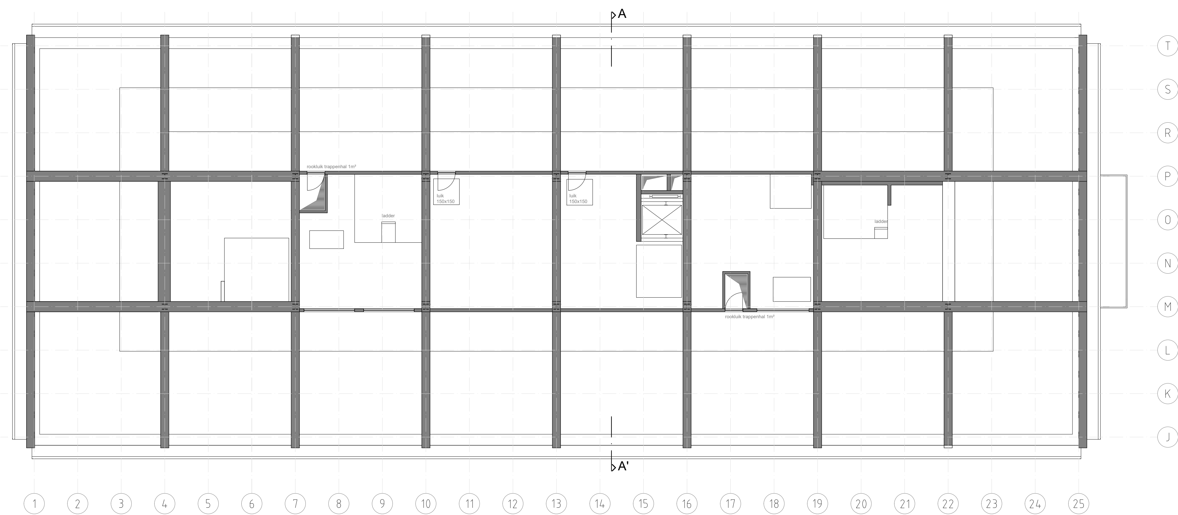
GRONDPLAN VERDIEPING 14
