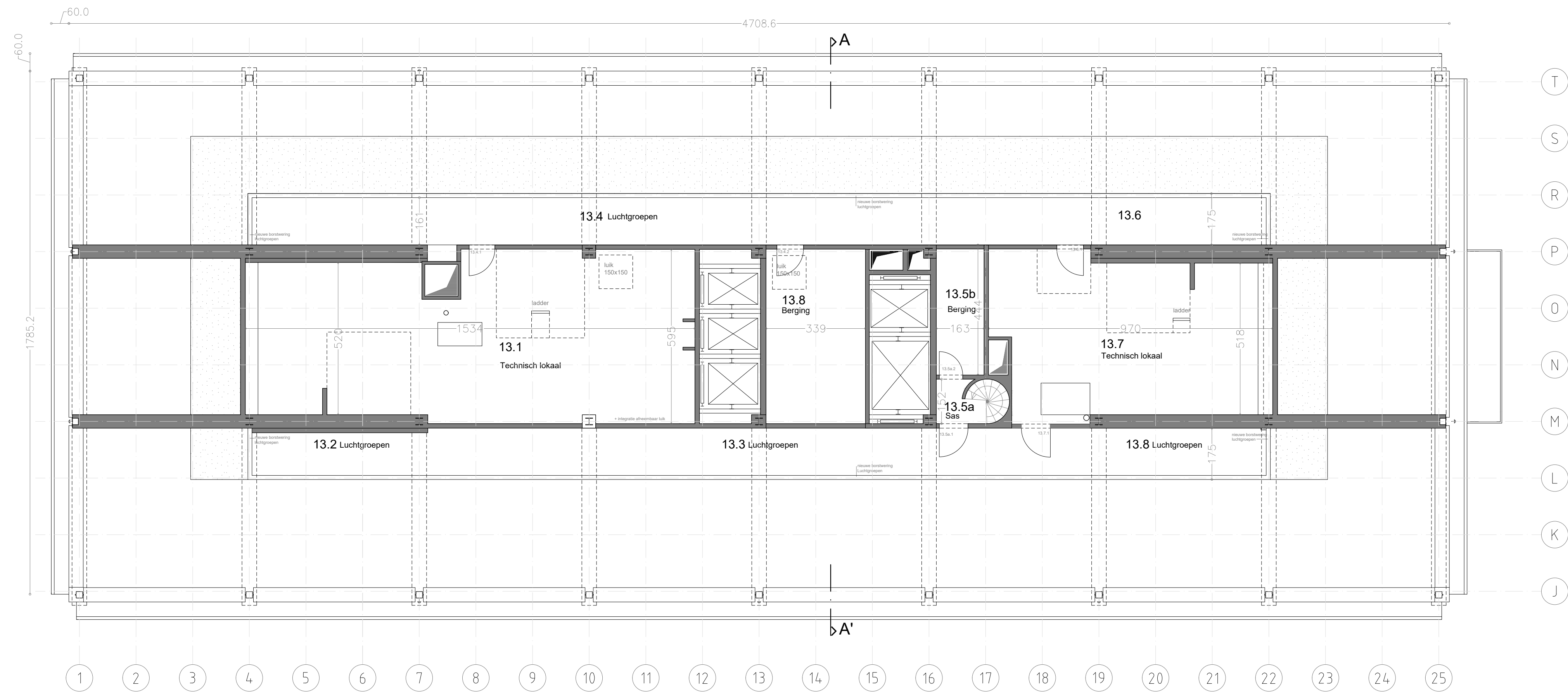
GRONDPLAN VERDIEPING 13
