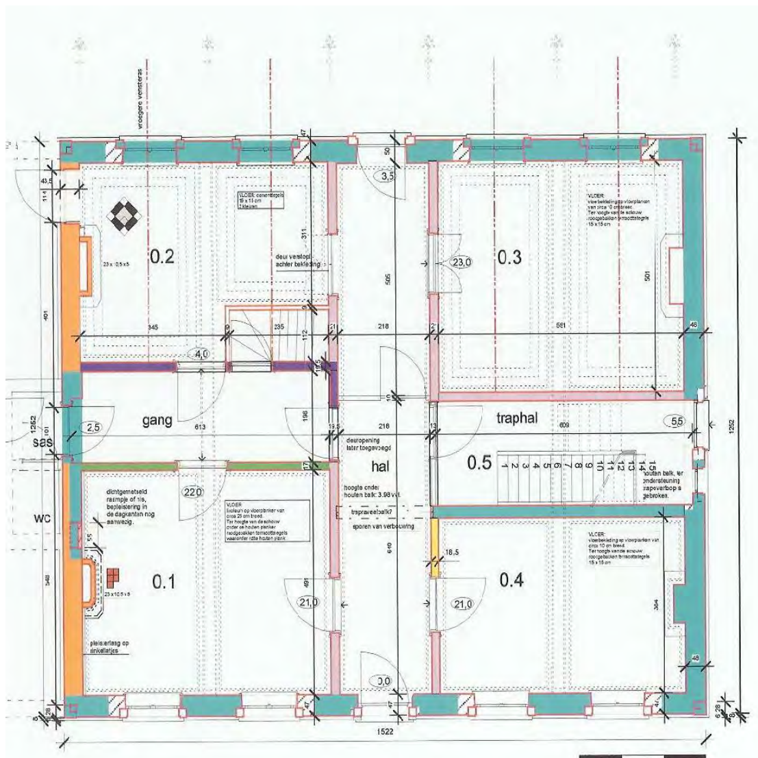
Afbeelding 56: grondplan gelijkvloers met nummering van de lokalen en kleuraanduiding van de baksteentypes. (eigen tekening, zie onder rubriek plannen, Deel A.3.)
