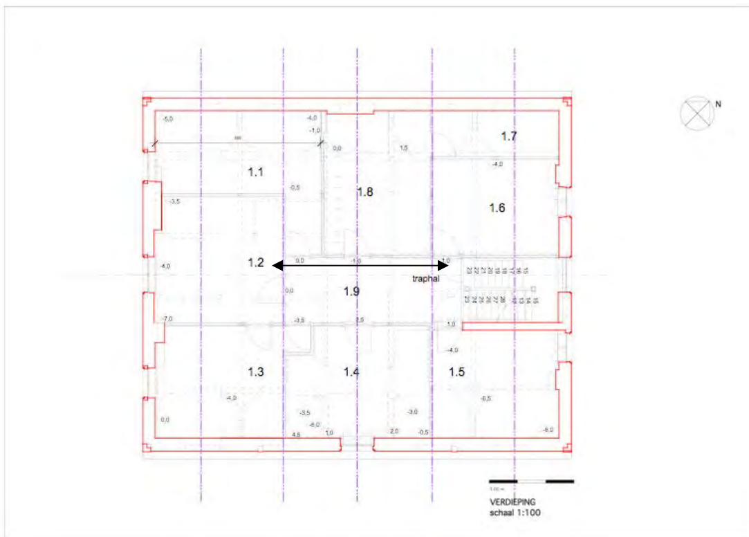
Afbeelding 53: Grondplan verdieping pastorie van Meuzegem. 72
