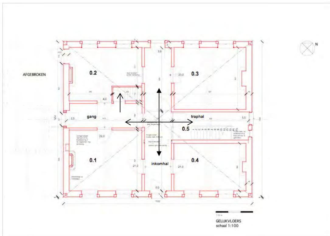
Afbeelding 52: Grondplan gelijkvloers pastorie van Meuzegem. 71
