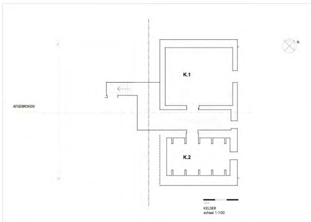
Afbeelding 51: Kelderplan pastorie van Meuzegem. 69
