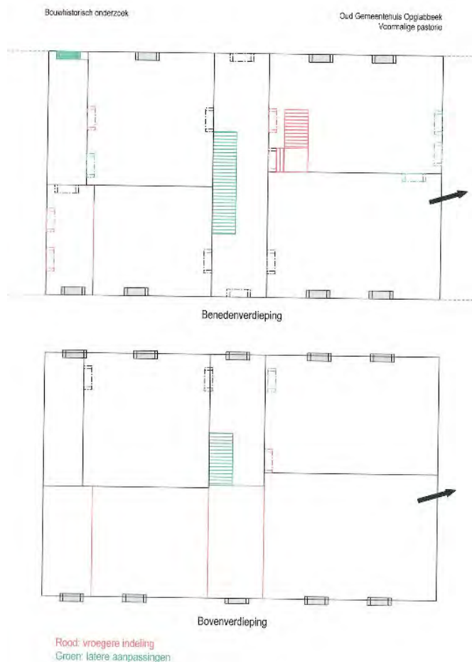
Afbeelding 50: Grondplan pastorie van Opglabbeek. 66
