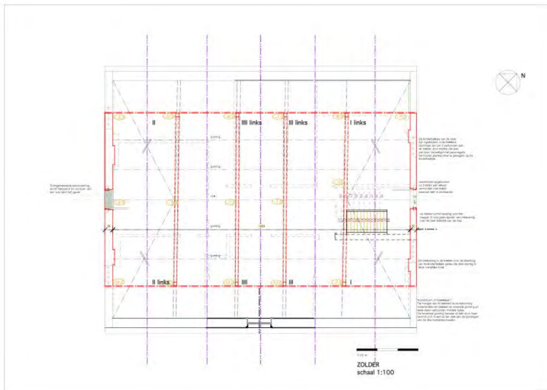
Afbeelding 54: Grondplan zolderverdieping pastorie van Meuzegem. 73
