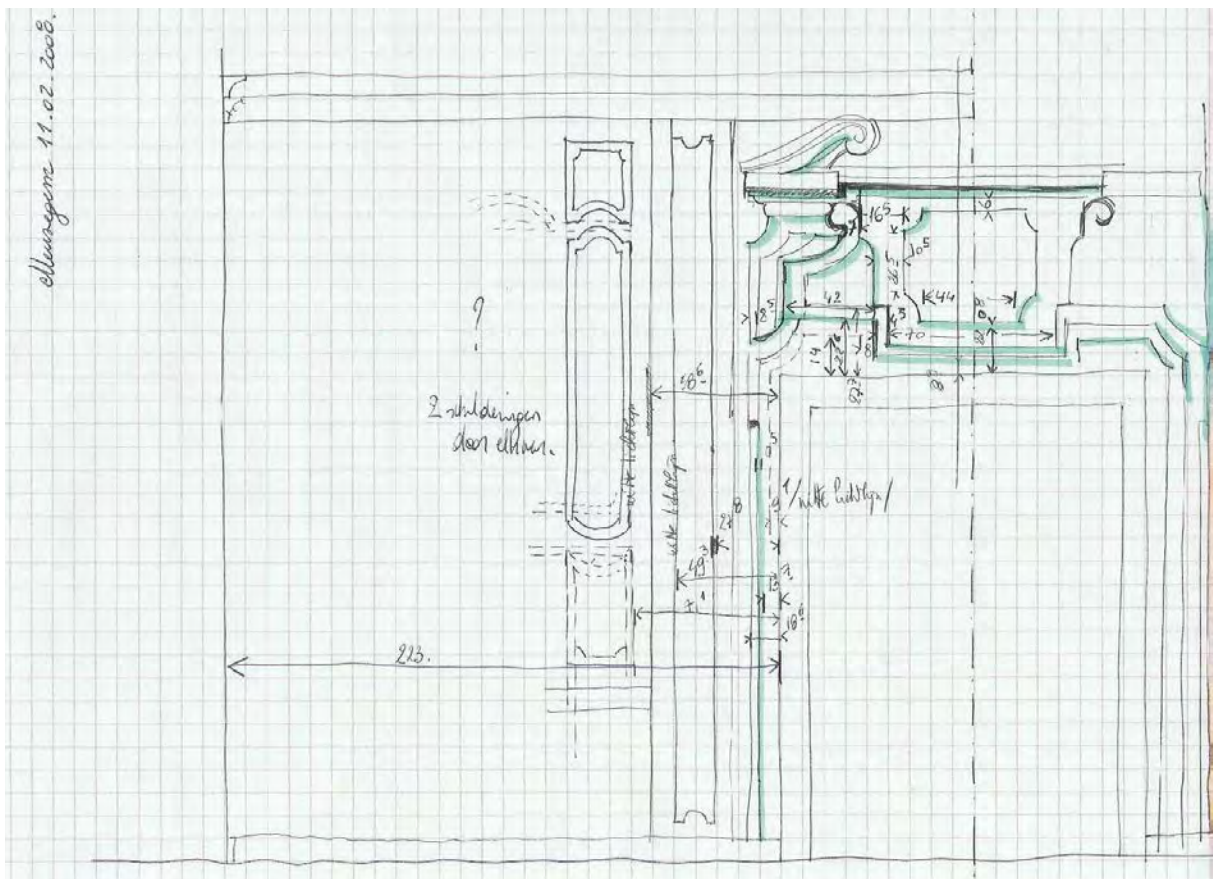
Afbeelding 47j: opmeting geschilderde kaders met schaduwwerking. Wand ZW, fronton boven de deur. Links van de deur is te zien hoe de schilderijen werden aangepast en overschilderd. 108
