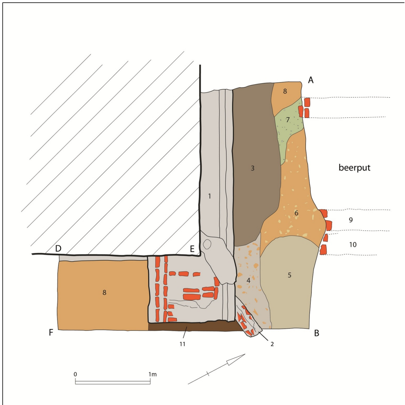
Fig. 15: sporenplan van de werkput: 1: funderingsconstructie uit baksteen en cement; 2: bakstenen ondersteuning onder 1; 3: funderingsleuf van 1; 4: grijs gele opvullingslaag; 5: geel grijze zandlemige opvullingslaag; 6: geelbruine lemige opvullingslaag met talrijke oranje leembrokken; 7: groene kleiige opvullingslaag; 8: vaste zandlemige bodem; 9: bakstenen wand van de beerput; 10: vernieuwing van de wand van de beerput; 11: bouwvoor.
