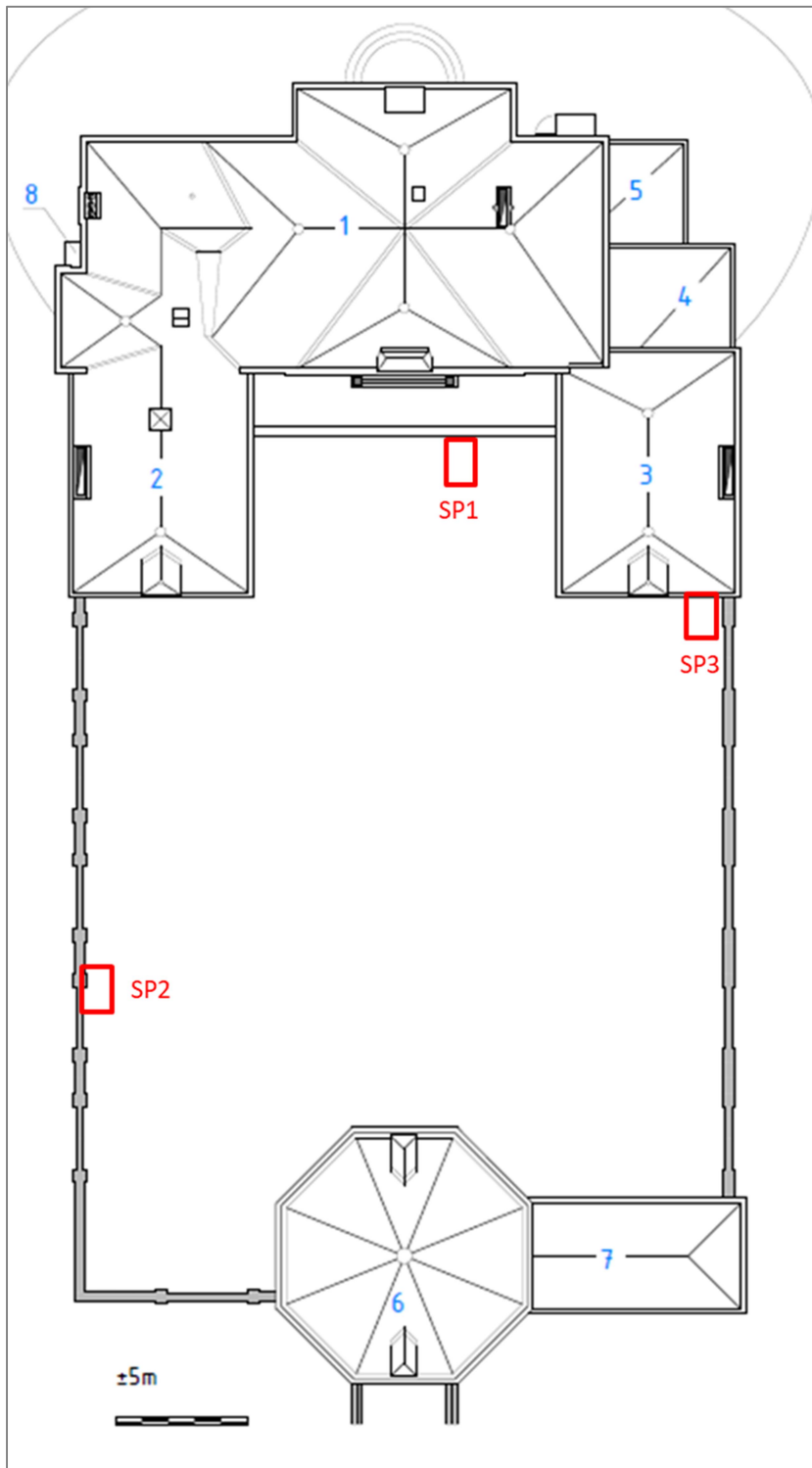
Figuur 1. Aalst Kasteel Ter Linden. Ligging sonderingsputten op het binnenplein. (Grondplan: Monumentenwacht)
