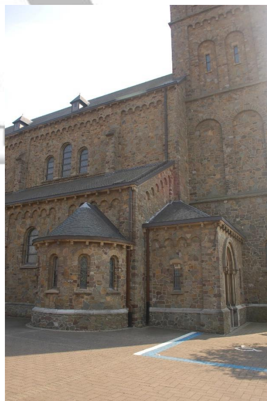
Situering: Veldwezelt | Sint Lambertuskerk. Beschrijving: Foto 6 | Algemene zichten | Extérieur. Bron: Architectenburo Erik Martens & Partners bvba | 2020.
