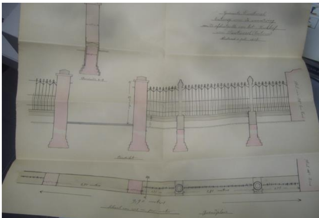
Figuur 2.2-43: Ontwerp afsluitgrille (1917) – Foto Gemeentearchief Wuustwezel
