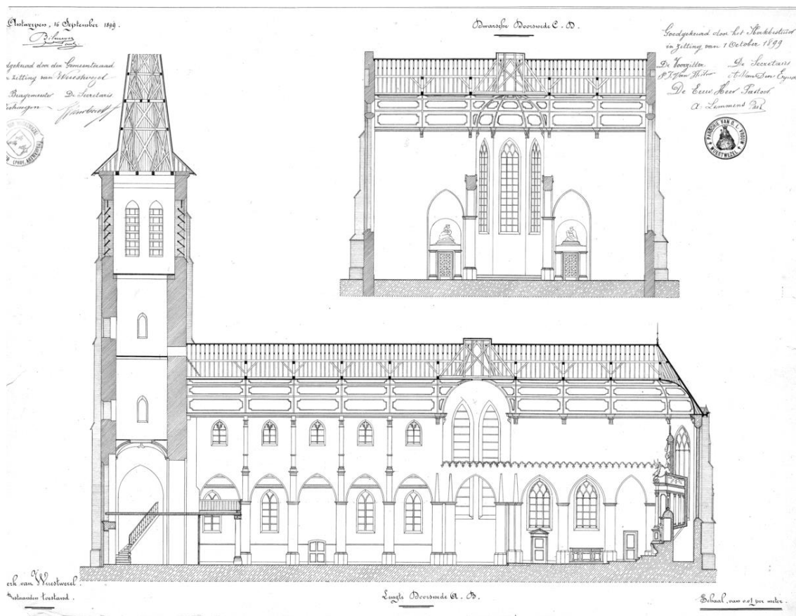
Figuur 2.2-4: Plan van bestaande toestand, 1899, Bilmeyer, RAA, PAA642
