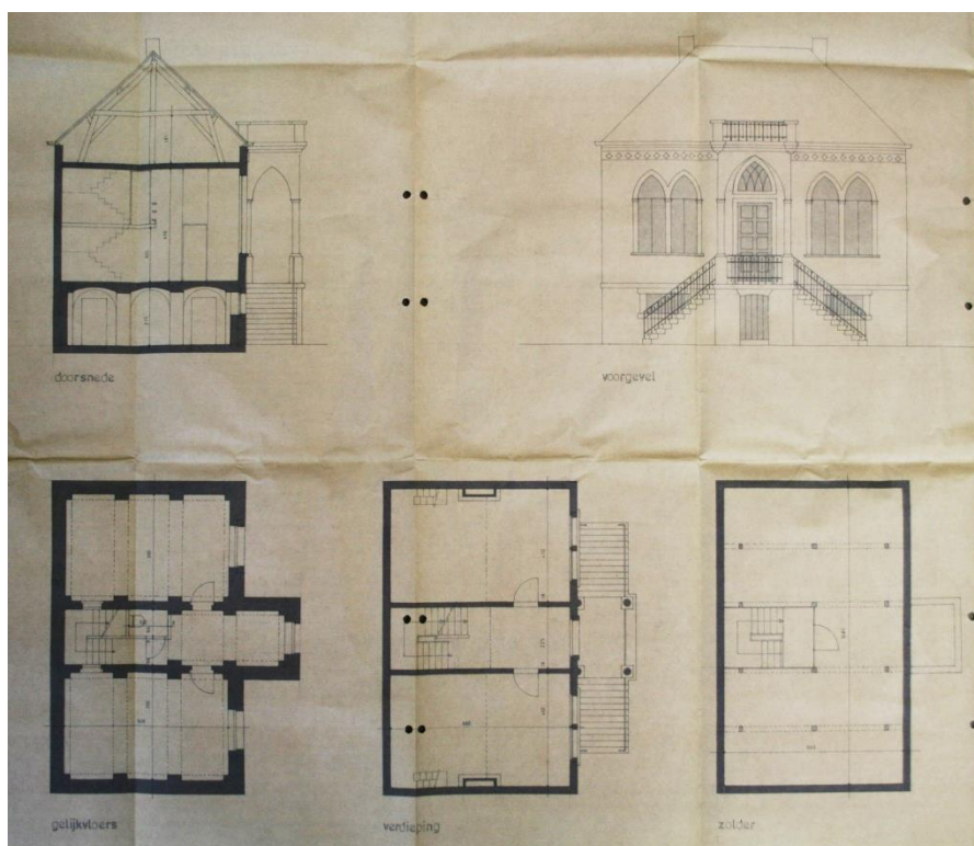
Figuur 2.2-18: Plan van een bestaande toestand van het oud gemeentehuis, Wesalia II
