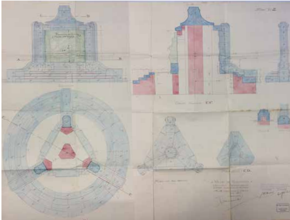
Afbeelding 8. Ontwerpplan van het monument door Emiel van Averbek. (© ARA)
