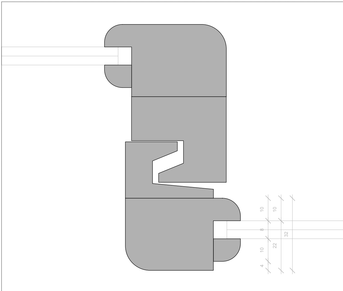
NIEUWE TOESTAND met gelaagd glas (4 mm - coating - 4 mm) (principeschets)
