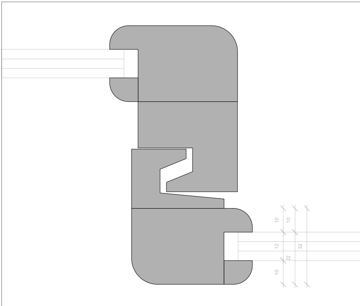
NIEUWE TOESTAND met dunne dubbele beglazing (4 mm - 4 mm spouw - 4 mm) (principeschets)
