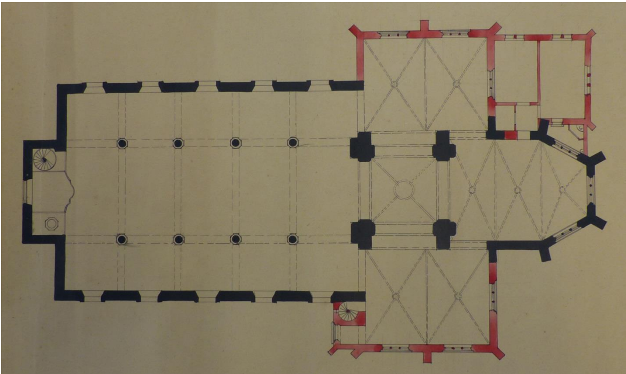
Figuur xi Grondplan (Bron: SAA: MAK Nieuwerkerken 29.)
