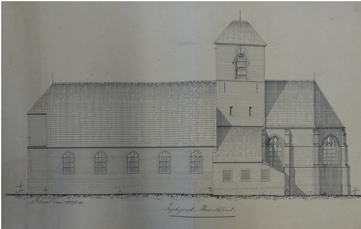
Figuur iii Zijgevel, zuidkant (Bron: SAA: MAK Nieuwerkerken 21.)
