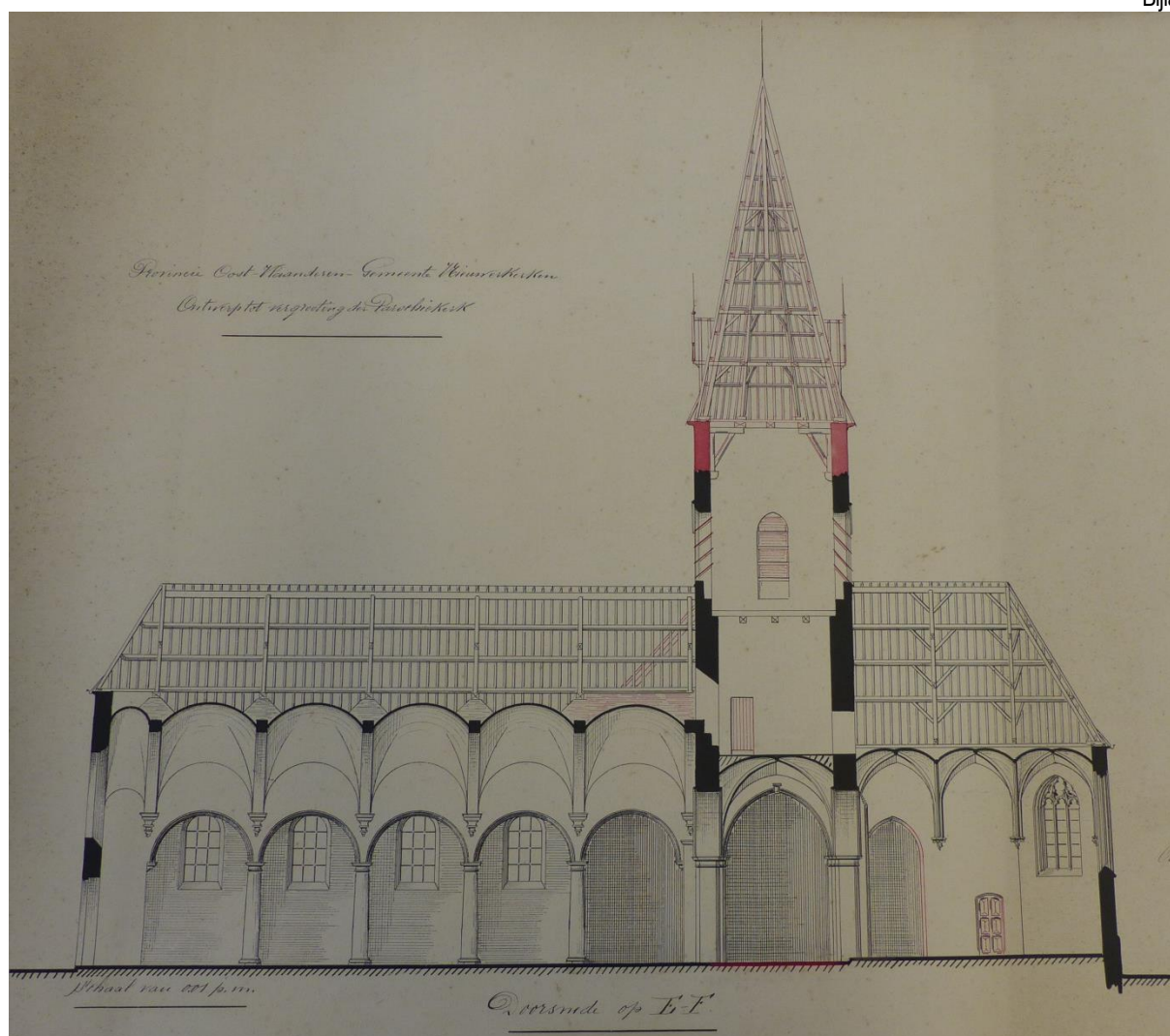
Figuur xiii Doorsnede EF (Bron: SAA: MAK Nieuwerkerken 30.)
