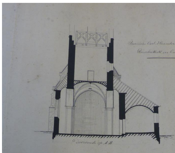
Figuur v Doorsnede AB en CD (Bron: SAA: MAK Nieuwerkerken 22.)
