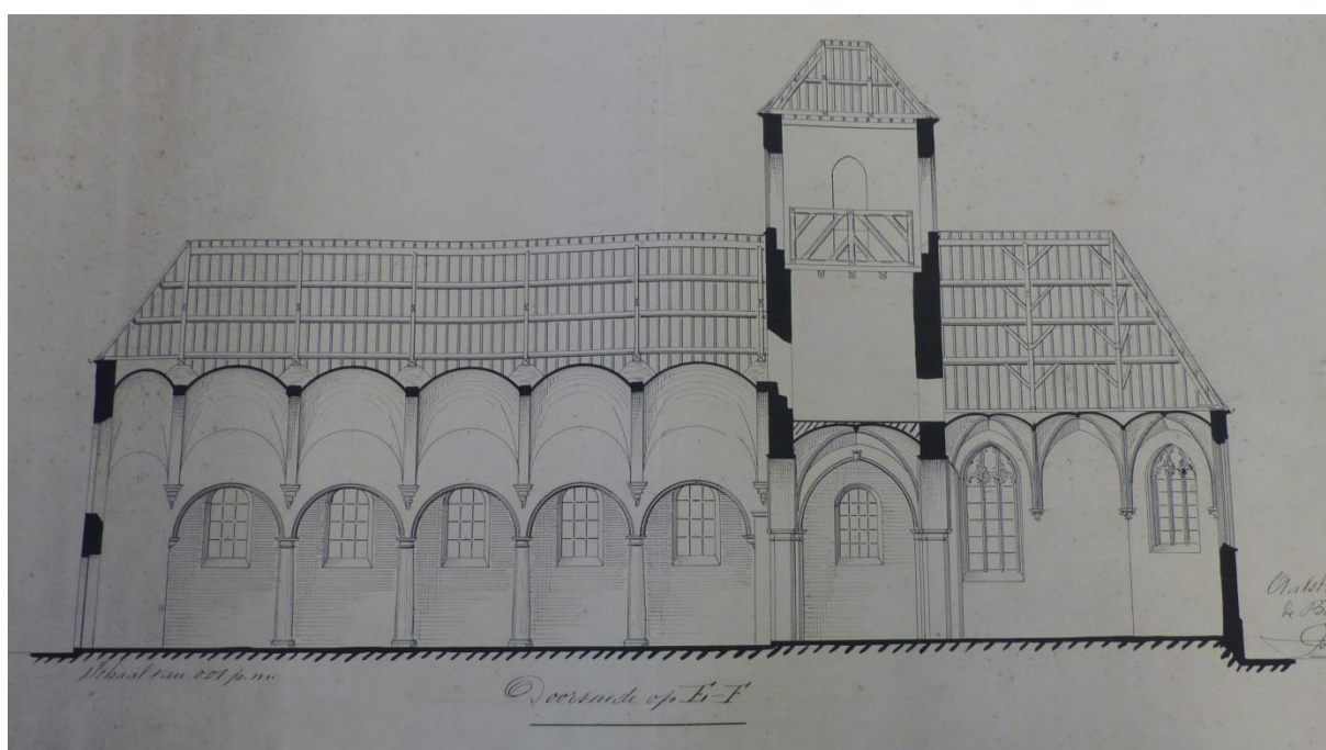
Figuur vi Doorsnede EF (Bron: SAA: MAK Nieuwerkerken 23.)
