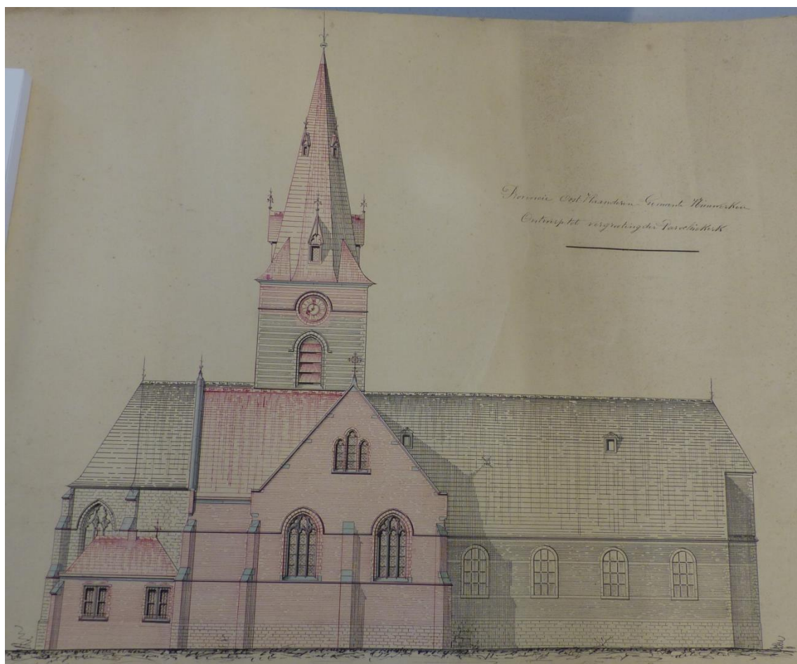
Figuur ix Zijgevel noordkant (Bron: SAA: MAK Nieuwerkerken 27.)
