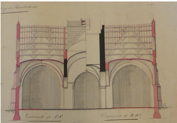
Figuur xii Doorsnede AB en CD (Bron: SAA: MAK Nieuwerkerken 29.)
