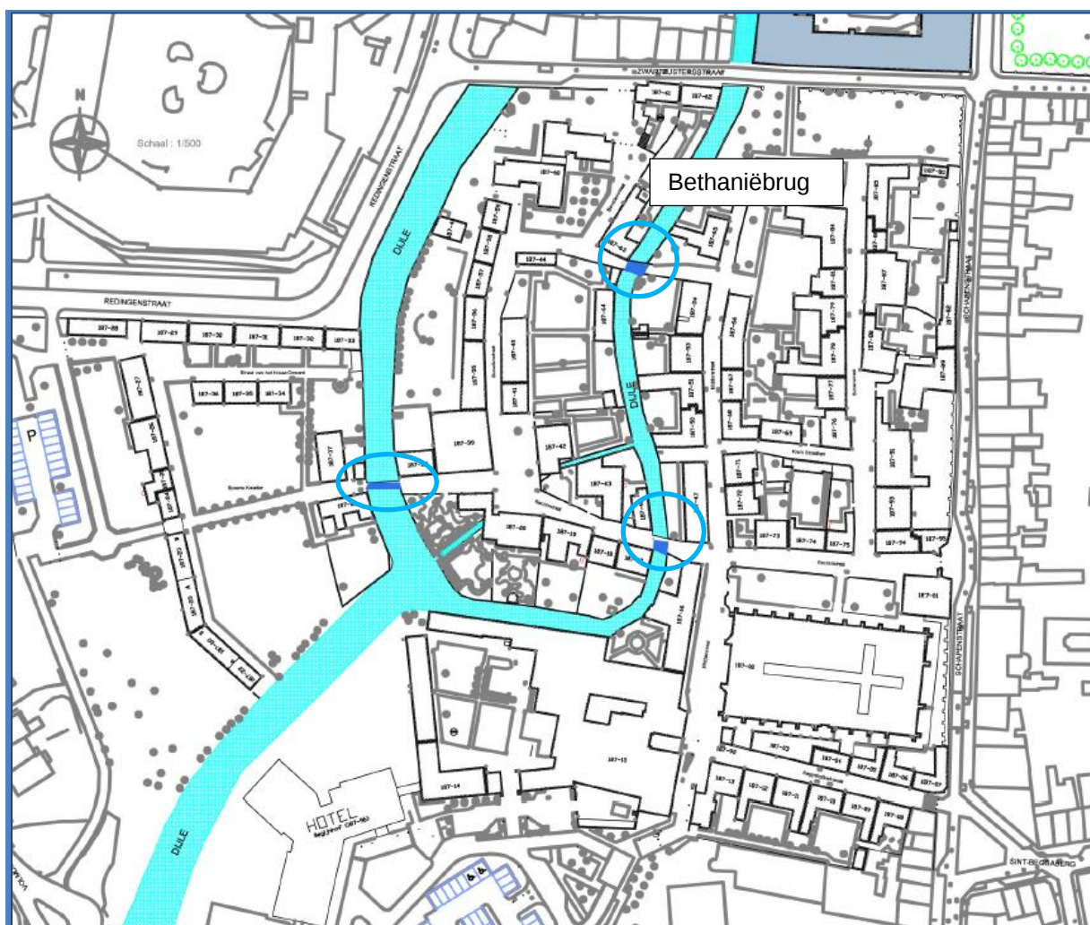
1 – Grondplan met aanduiding bruggen in het Groot Begijnhof Leuven, brug over de Kleine Dijle in de Rechtstraat, brug over de Dijle in de Rechtstraat en brug over de Kleine Dijle aan het Convent van Bethanië, Technische Diensten KU Leuven.
